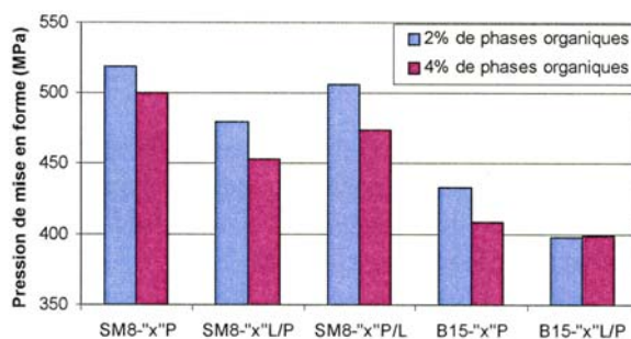
Figure 4. Pression de mise en forme obtenue pour chacune des poudres d'alumine testées en CGV.
