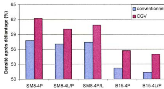
Figure 8. Densité après déliantage des comprimés conventionnels et CGV
