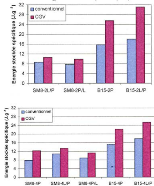
Figure 5. Energie stockée spécifique à 400 MPa pour chacune des poudres et des méthodes de mise en forme.
