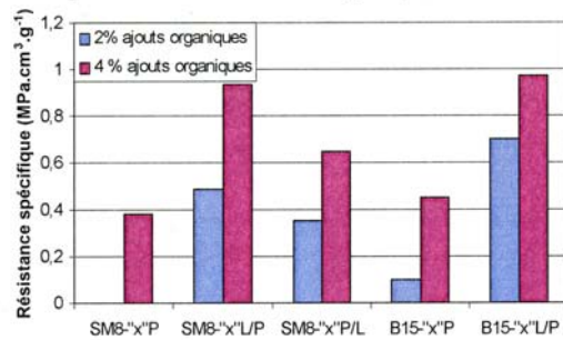
Figure 6. Résistance mécanique spécifique des comprimés élaborés conventionnellement
