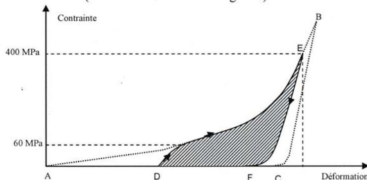
Figure 2. Représentation des zones de travail de compression
