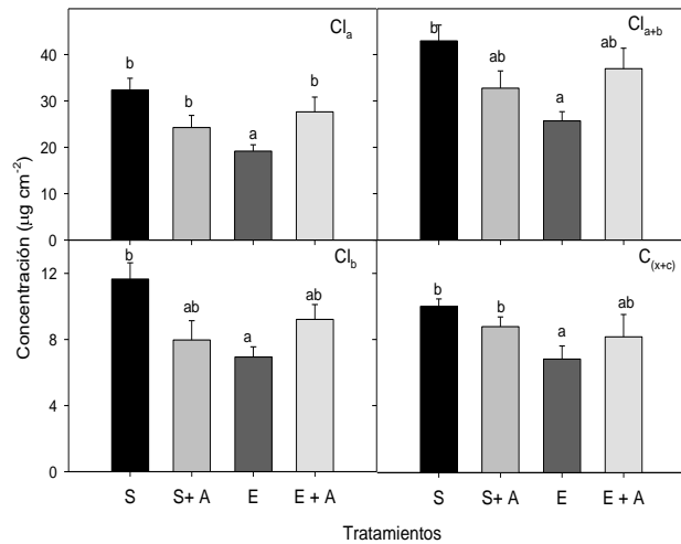
Figura 4. Concentración de clorofila a ( Cl_a ), clorofila b ( Cl_b ), clorofila total ( Cl_{a+b} ) y carotenoides totales ( C_{x+c} ), en hojas de los árboles de cacao (OC-61) en los tratamientos S, S+A, E y E+A. Los valores representados son los promedios \pm error estándar ( n = 5 ). Las diferentes letras indican diferencias significativas ( p < 0.05 ) entre tratamientos.
