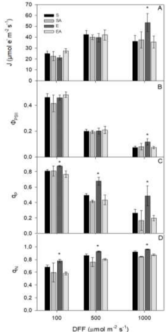
Figura 3. Transporte total de electrones (J), Eficiencia cuántica relativa del PSII ( \Phi_{PSII} ), Coeficiente de extinción fotoquímica ( q_P ) y Coeficiente de extinción no fotoquímica ( q_N ) determinados a tres diferentes densidades de flujo de fotones (DFF) en hojas provenientes de los árboles de cacao (OC-61) de los tratamientos S, S+A, E y E+A. Los asteriscos indican diferencias significativas entre tratamientos. Los valores representados son los promedios \pm error estándar (n = 4).
