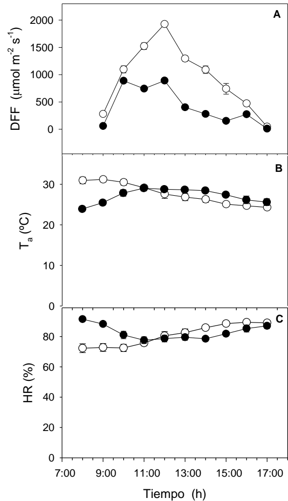
Figura 1. Curso diario de las variables microclimáticas: A. Densidad de flujo fotónico; B. Temperatura del aire; C. Humedad relativa. Las medidas realizadas en las dos diferentes condiciones del cultivo de cacao OC-61 a plena exposición solar (E, círculos abiertos) y en sombra (S, círculos cerrados). Los valores representados son los promedios \pm error estándar de datos obtenidos durante un mes ( n = 30 ).
