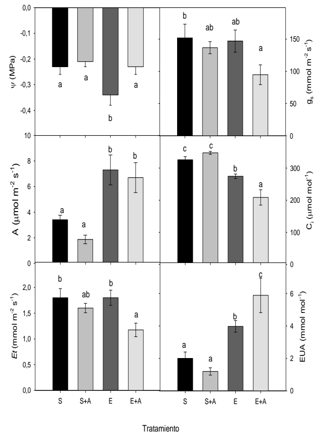
Figura 2. Potencial hídrico ( \Psi ), tasa fotosintética ( A ), transpiración ( Et ), conductancia estomática ( g_s ), concentración intercelular de \text{CO}_2 ( C_i ), eficiencia del uso de agua (EUA) en los árboles de cacao (OC-61) con los tratamientos: sombra (S), sombra con auto sombreado (S+A), expuesto (E), y expuesto con autosombreado (E+A). Los valores representados son los promedios \pm error estándar ( n = 5 ). Las diferentes letras indican diferencias significativas ( p < 0.05 ) entre tratamientos.
