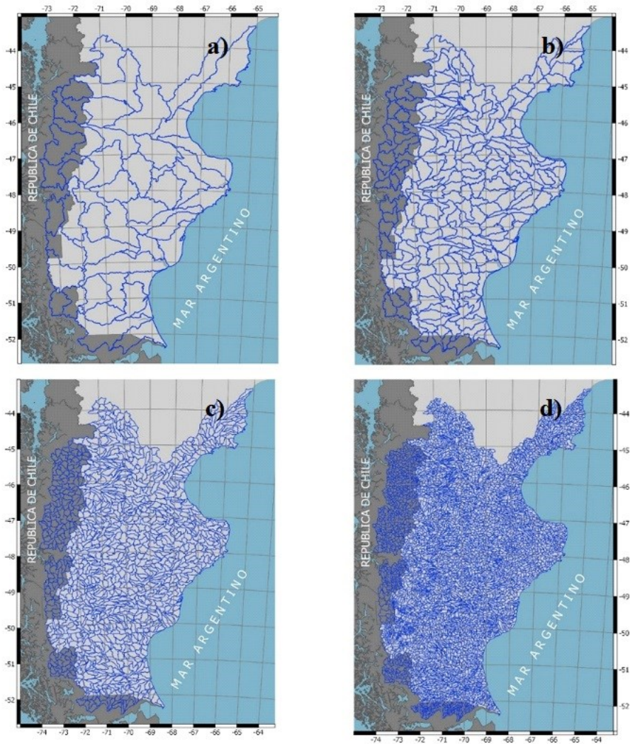
Figura 2. Mapa de UH desarrolladas para la Patagonia Austral continental en diferentes niveles de anidación (a) nivel 2, SH; (b) nivel 3, CC; (c) nivel 4, SC; y nivel 5, MC.
