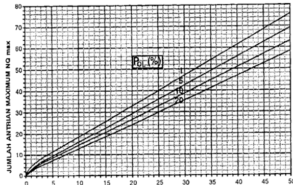
Gambar 4 Jumlah Antrian Maximum (NQ)
