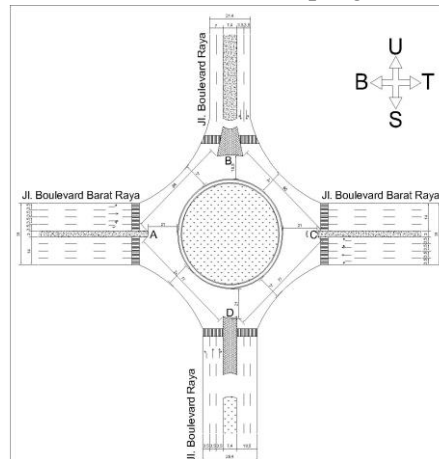
Gambar 3. Sketsa Bundaran Kelapa Gading
