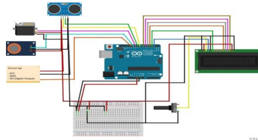
Gambar 9. Perancangan Sistem
