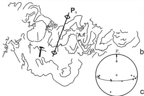
Figura 11: a) Afloramiento de volcanitas plegadas correspondientes a la sucesión arenigiana en Punta Pétrea ( 27^{\circ}47'40'' - 68^{\circ}02'47'' S). b) Esquema donde se detallan las estructuras que caracterizan este afloramiento. c) Datos estructurales que permiten definir al plegamiento P_2 en este afloramiento.
