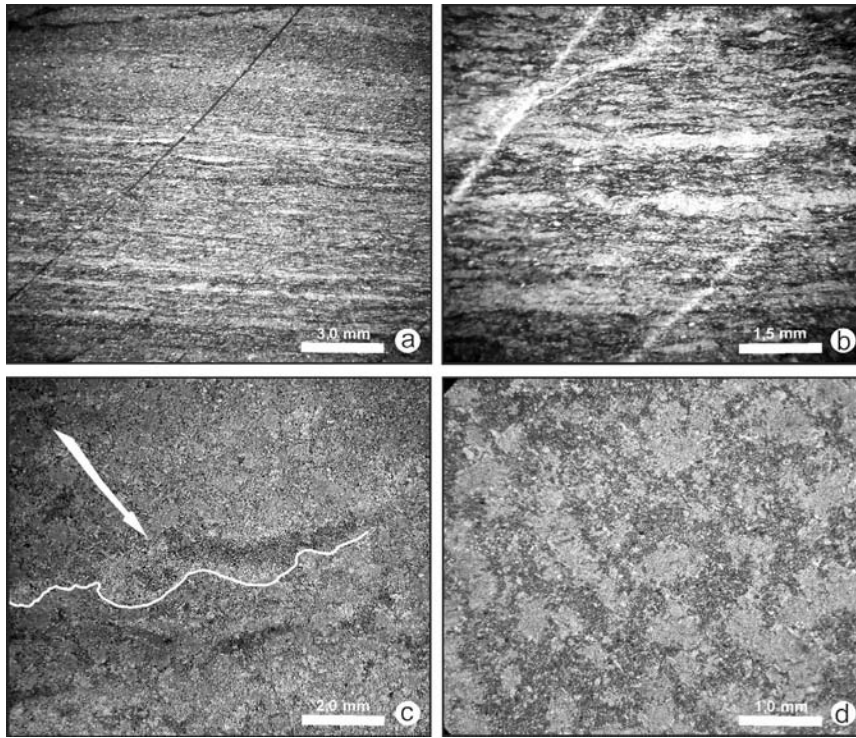
Figura 5: Fotomicrografías. a) y b) Clivaje anastomosado en lutitas, donde la foliación S1 se orienta según 115^{\circ} 50^{\circ} (Polarizador X). c) Limolita con lentes cuarzosos plegados (Polarizador X). d) Motas de mica blanca en limolita (Polarizador X).
