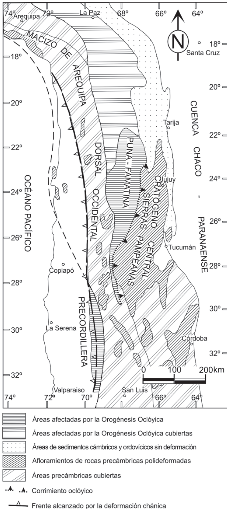
Figura 1: Mapa geológico esquemático del Cinturón Oclóyico y de su marco regional (modificado de Mon 1992). 1) Macizo de Arequipa; 2) Dorsal Occidental; 3) Precordillera; 4) Puna - Famatina; 5) Cratígeno Central (Sierras Pampeanas); 6) Cuenca Chaco - Paranaense.
