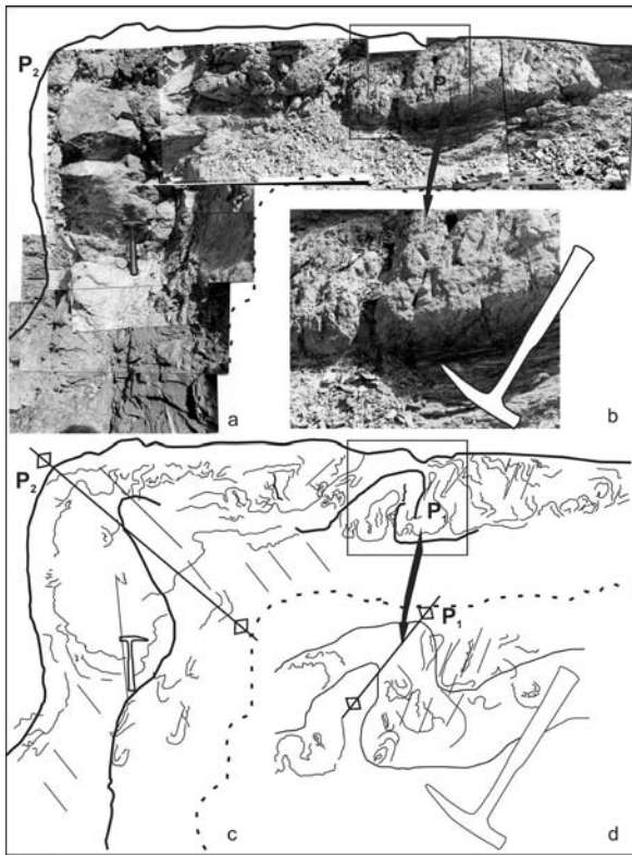
Figura 9: Detalle del afloramiento (27°42'10.2" S - 67°57'20.5" O). a) y b) Limolitas y volcanitas deformadas según dos episodios de plegamiento superpuestos, P 1 y P 2 . c) y d) Detalle de los niveles epiclásticos plegados y el clivaje de plano axial correspondiente a P 1 .
