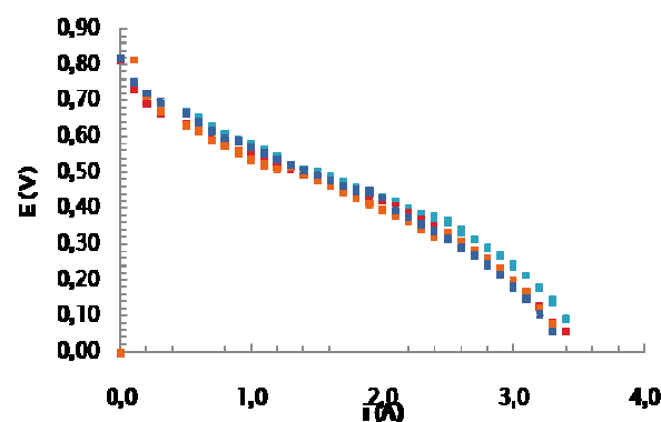
Figura 3. Desempeño del prototipo II. E vs i. Tcelda= 45° C, T humidificación: 50 °C. Relación de caudales 1:1.
