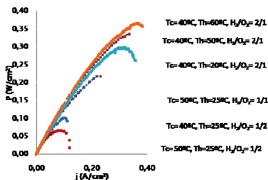
Figura 1. Densidad de potencia vs densidad de corriente para algunas de las condiciones de operación evaluadas.
