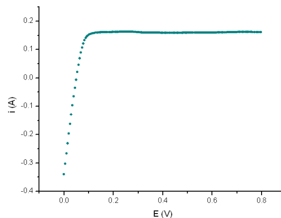
Figura 2. Corriente crossover de H 2 . LSV utilizando como electrodo de trabajo el cátodo, v= 4 mV/s. Relación de caudales N 2 /H 2 = 5/3
