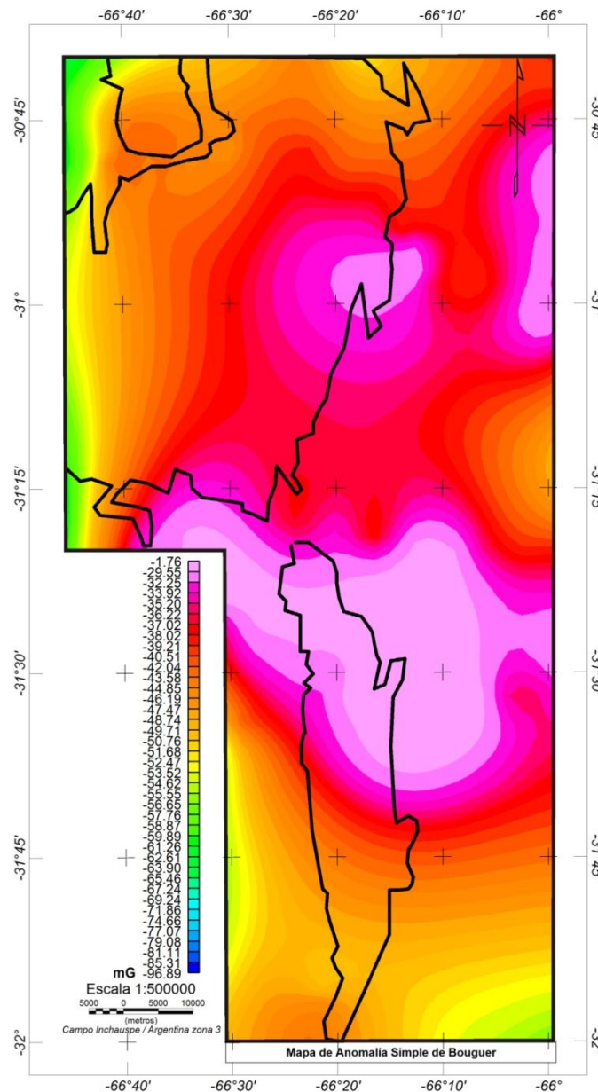
Figura 14. Mapa de Anomalia Simple de Bouguer.
