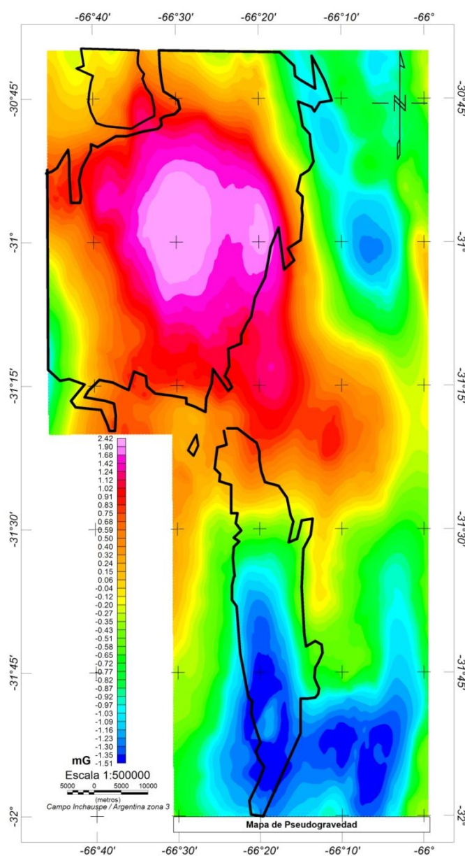
Figura 13. Mapa de Pseudogravedad.
