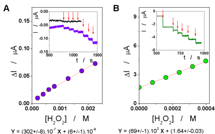
Figura 6: (a) Curva de calibración obtenida para electrodos modificados por autoensamblado. Inserto: detección amperométrica para alícuotas de 30 \mu\text{L} y 60 \mu\text{L} de H 2 O 2 (0,1 M) en PBS (pH 7) para GCE (negro) y GCE modificado por autoensamblado (violeta). (b) Curva de calibración obtenida para electrodos modificados por casting , por adición de estándar. Inserto: detección amperométrica para alícuotas de 20 \mu\text{L} de muestra (0,3 M) y agregados posteriores de 20 \mu\text{L} de soluciones de H 2 O 2 (0,1 M) en PBS (pH 7).
