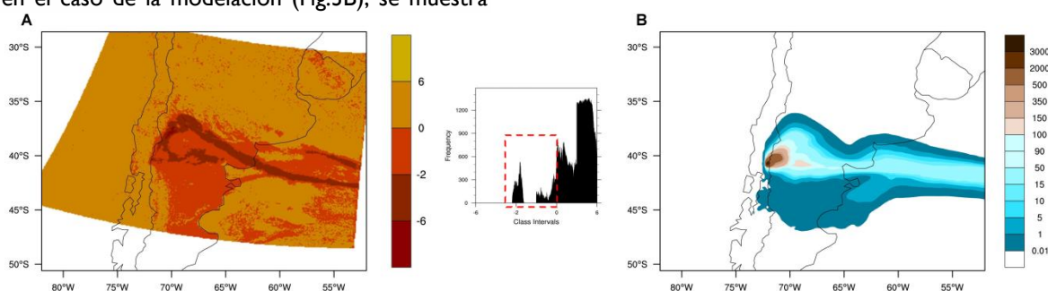
Figura 3: Comparación cualitativa para el 6 de junio de 2011 a las 14:15 UTC entre la discriminación de aerosoles volcánicos utilizando el método de Prata (izquierda) y entre la columna de ceniza volcánica (en g/m^2 ) simulada con FALL3D (derecha). Se muestra también el correspondiente histograma de frecuencias determinado por Prata.
