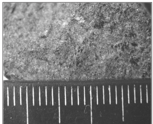
FIGURA 12 • MENA MAGMÁTICA.
