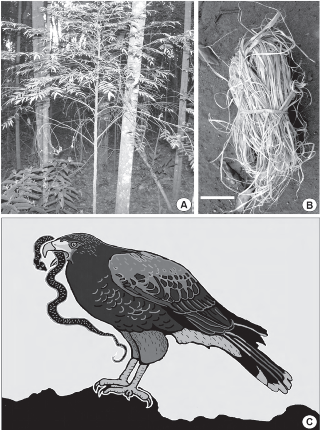
Fig. 1. A: Ejemplares juveniles de una población de Xylopi brasiliensis (Annonaceae) . B: Tejido fibroso extraído manualmente de su floema secundario (escala 5 cm). C: Representación de Parabuteo unicinctus (Falconidae) devorando una culebra.
