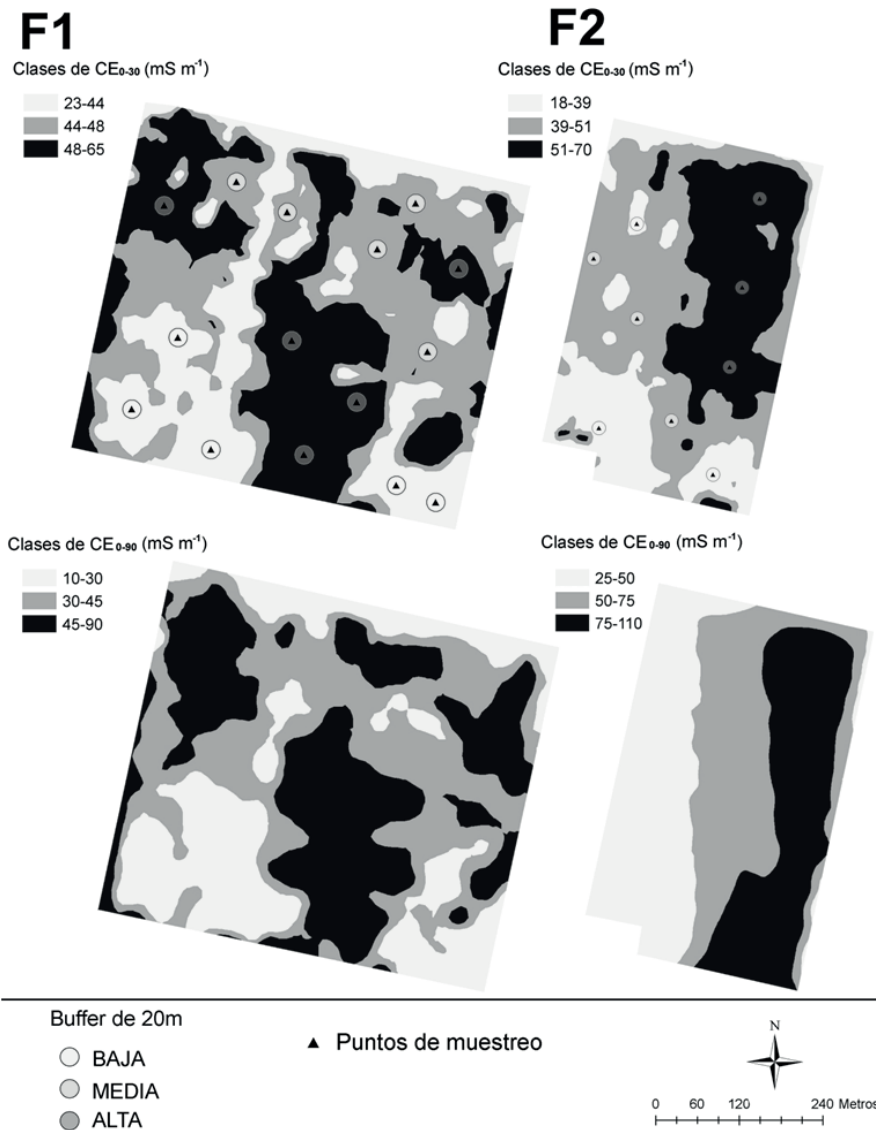
Figura 3. Mapa de conductividad eléctrica aparente ( CE_a ) para cada lote. Figure 3. Apparent electrical conductivity ( CE_a ) map for each field.
