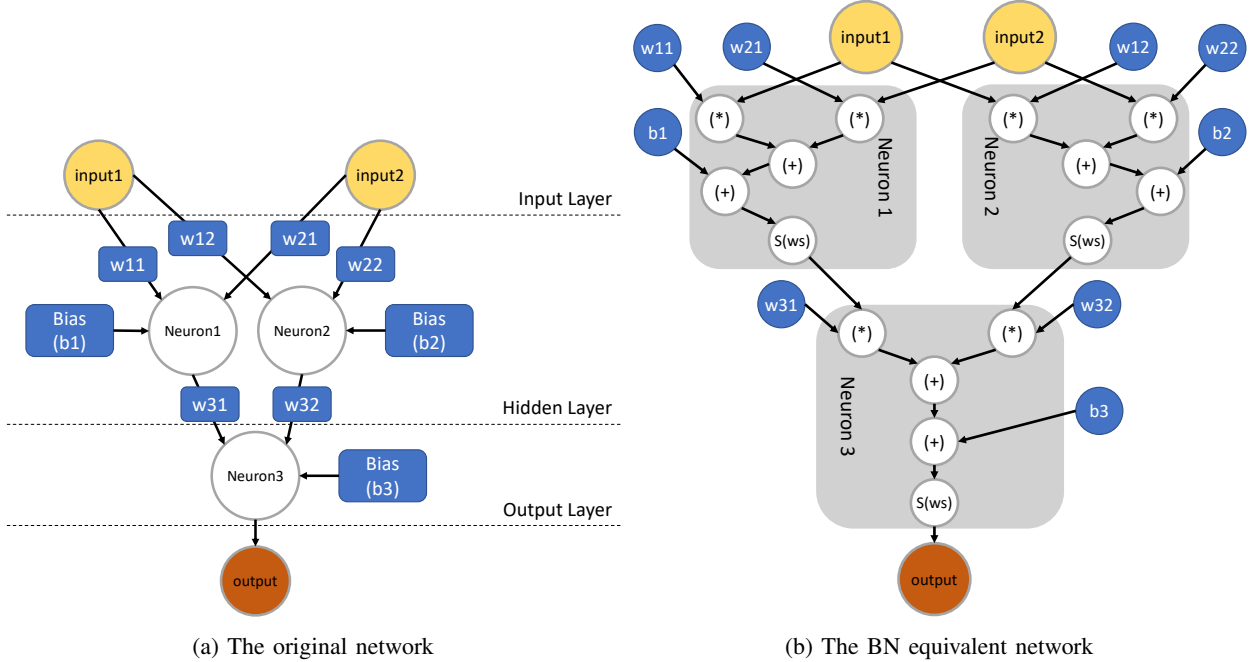
Fig. 2: XOR network
