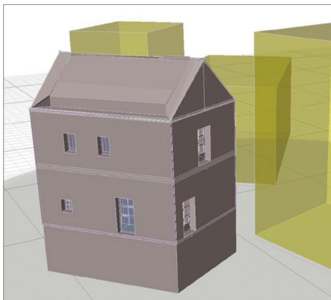
Figura 6. Vista tridimensionale del modello dell'edificio (Termolog).
