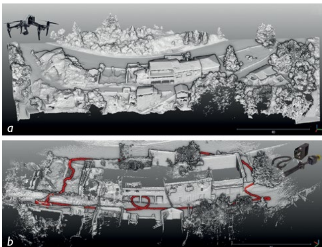
Figura 4. Confronto tra modelli: (a) nuvola DSM del volo fotogrammetrico UAV; (b) mappatura 3D da ZEBI mobile mapping system con visibilità della traiettoria percorsa, in rosso.
