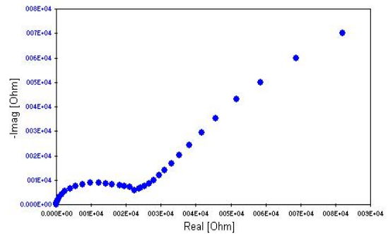
Figura 7. Diagrama de Nyquist para el segundo modelo
