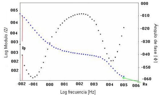
Figura 5. Diagrama de Bode para el segundo modelo
