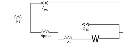
Figura 6. Circuito equivalente para el segundo modelo
