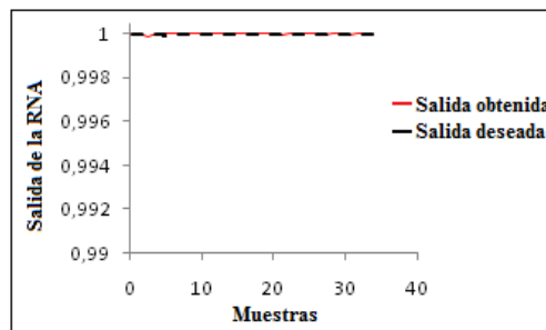
Figura 7. Respuesta del caso 3 en operación normal.
