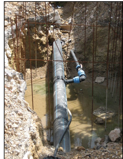
Figure 3 : Le réseau d'eau potable de Chekka. (Photo : C. Féré)
