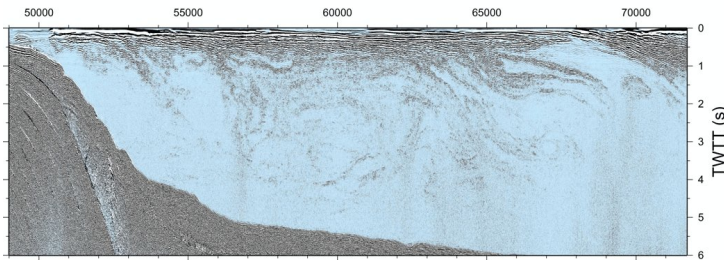
Fig. 2.6. Imagerie en réflexion sismique permettant de visualiser les différentes masses d'eau par les différents échos renvoyés après une détonation [23].
