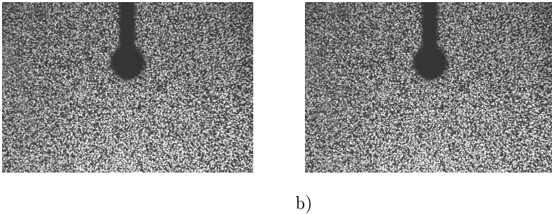
Fig. 3.9. Images utilisées pour la mesure des gradients de densité par strioscopie synthétique. a) Image de référence. b) Image en présence des ondes. La différence est imperceptible à l'œil mais permet en utilisant des algorithmes de PIV de reconstruire le champ de densité.
