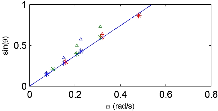
Fig. 8.23. Relation de dispersion pour les différents harmoniques des cas A, B et C. Les étoiles marquent les modes propagatifs vérifiant la loi théorique \omega = N \sin \theta . Les triangles représentent les modes forcés mesurés dans la zone interne de réflexion et ne vérifiant pas la relation de dispersion.
