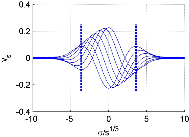
Fig. 4.3. Coupe transverse du profil auto-similaire de vitesse établi par Thomas et Stevenson [44]. Les différentes courbes correspondent aux phases 0, \pi/6, 2\pi/6, 3\pi/6, 4\pi/6, 5\pi/6 et 6\pi/6 de l'onde. Les traits en pointillé définissent la largeur du faisceau comme la distance séparant à phase nulle les points de vitesse extrême.
