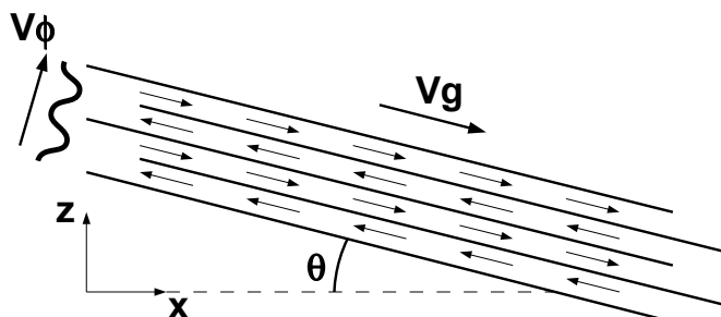
Fig. 1.2. Structure d'une onde interne. Le cisaillement de propagation vers le haut selon la vitesse de phase, tandis que le rayon progresse vers le bas selon la vitesse de groupe.
