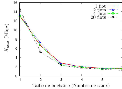
Figure 3. \bar{X}_{max} fonction du nombre de sauts
