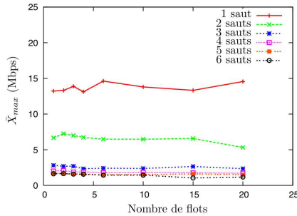
Figure 2. \bar{X}_{max} fonction du nombre de flots TCP
