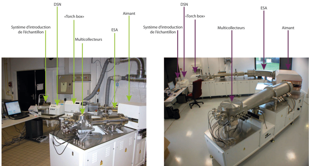
FIGURE 8.3.1: Organisation d'un Nu 500 (à gauche) et Nu 1700 (à droite). Photographie : Philippe Telouk. DSN = Desolvating nebuliser system. ESA=Electrostatic analyser
