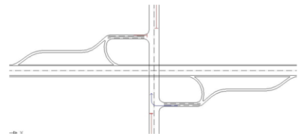
Gambar 7. Gambar Setting Fase pada Parclo B2 Modifikasi
