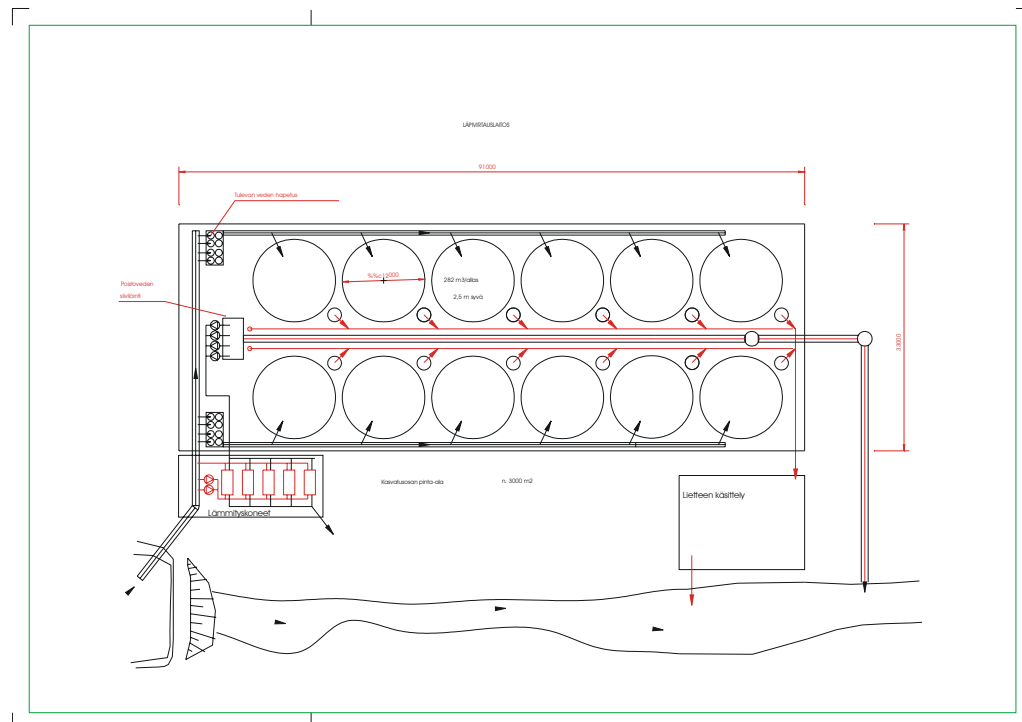
Kuva 3. Lämpivirtauslaitoksen rakenne.
