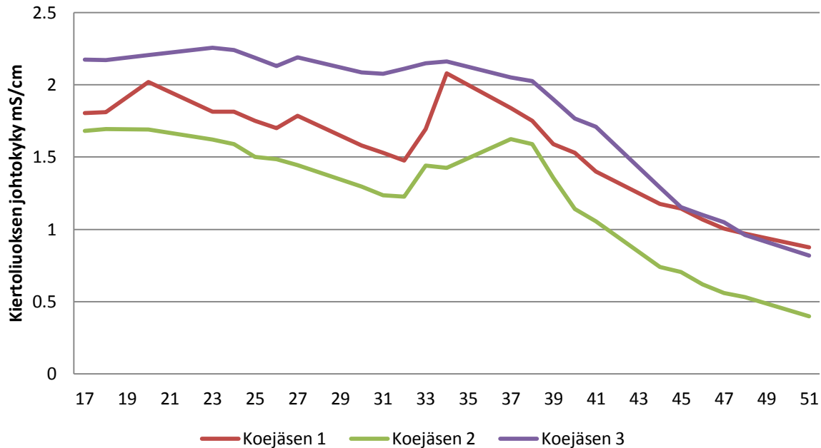
Kuva 2. Kiertoliuoksen johtokyky ( \text{mS cm}^{-1} ) eri koejäsenillä jääsalaatin kouruviljelyn aikana (vrk kylvöstä) kesällä.
