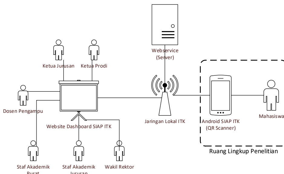
Gambar 1 Arsitektur SIAP ITK.
