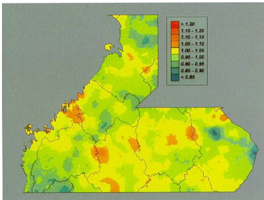
Kuva 2. a) Mäntyvaltaisten metsiköiden valtipituusboniteetti kangasmailla. b) Mäntyvaltaisten metsiköiden valtipituusboniteetti suhteessa yhtälöllä ennustettuun (taulukko 7, mänty).
