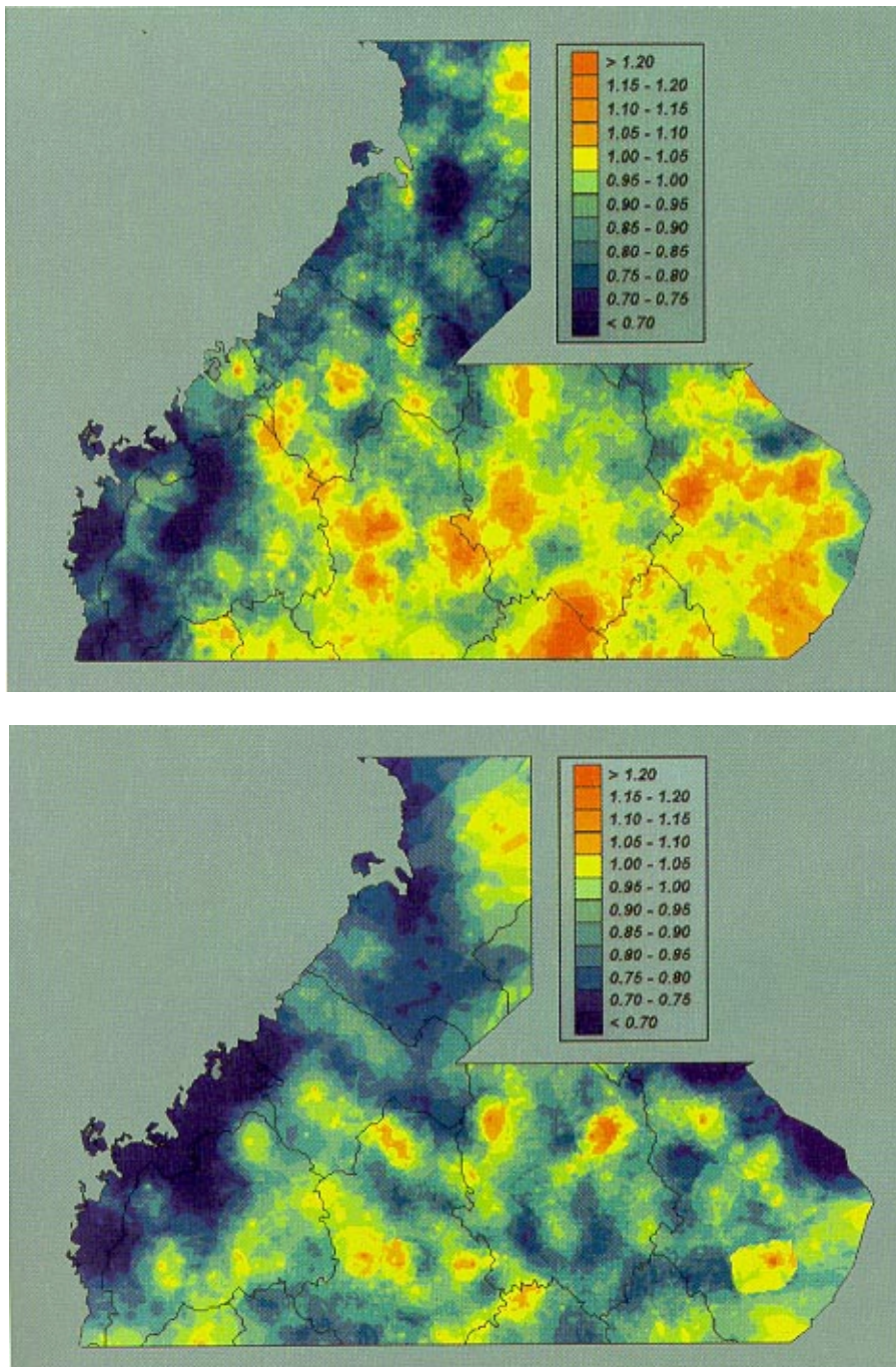
Kuva 6. Männiköiden (a) ja kuusikoiden (b) mitatun ja ennustetun tilavuuskasvun suhde (=tasokerroin). Kasvu ennustettiin Nyssösen ja Mielikäisen (1978) mallilla.
