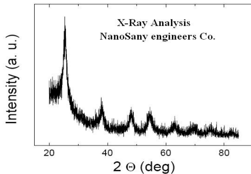
نمودار شماره ۱: XRD نانو ذره دی‌اکسید تیتانیوم
