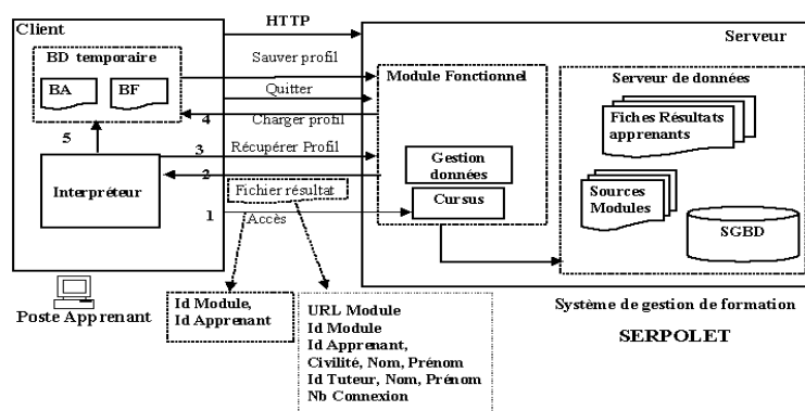
Figure 3. Déroulement d'un module et gestion des parcours dans SERPOLET
