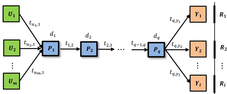
Gambar 1: Flow line dengan m input, q pemroses, l output, dan l waktu deadline [6].
