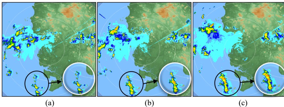
Gambar 4 Contoh kasus QLCS broken line di wilayah Pontianak tanggal 27 Mei 2019 pukul (a) 19.54 UTC, (b) 20.14 UTC, dan (c) 20.49 UTC
