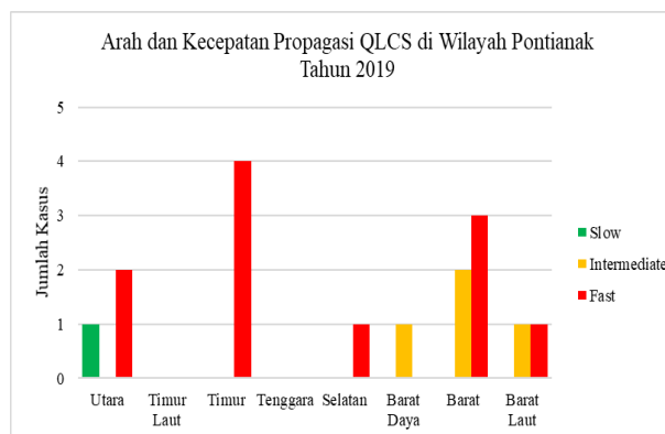
Gambar 7 Distribusi arah dan kecepatan propagasi sistem QLCS di wilayah Pontianak tahun 2019
