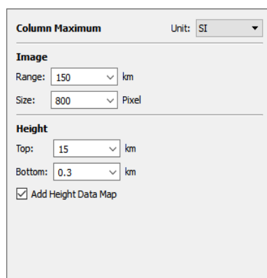
Gambar 1 Pengaturan produk CMAX
