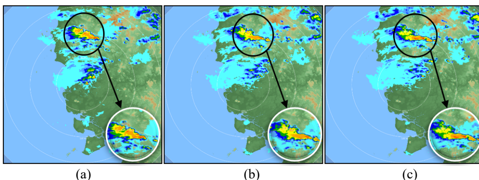
Gambar 5 Contoh kasus QLCS back building di wilayah Pontianak tanggal 07 Februari 2019 pukul (a) 09.36 UTC, (b) 09.51 UTC, dan (c) 09.56 UTC
