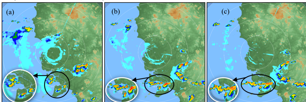
Gambar 6 Contoh kasus QLCS broken areal di wilayah Pontianak tanggal 26 September 2019 pukul (a) 09.17 UTC, (b) 09.52 UTC, dan (c) 10.07 UTC.
