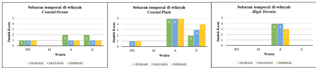
(a) (b) (c) Gambar 3 Sebaran temporal QLCS di wilayah (a) Coastal Ocean (CO), (b) Coastal Plain (CP), (c) High Terrain (HT) Pontianak Tahun 2019
