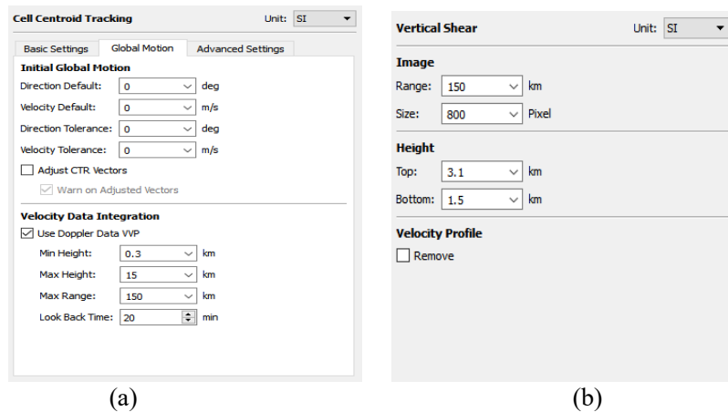
(a) (b) Gambar 2 Pengaturan produk (a) CTR dan (b) VSHEAR
