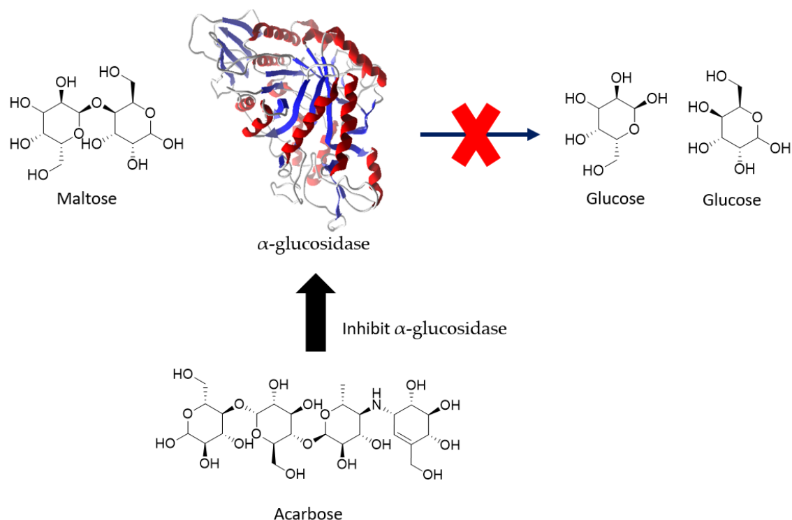
Gambar 4. Mekanisme Acarbose Menurunkan Gula Darah
