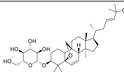
Momordicoside F1
