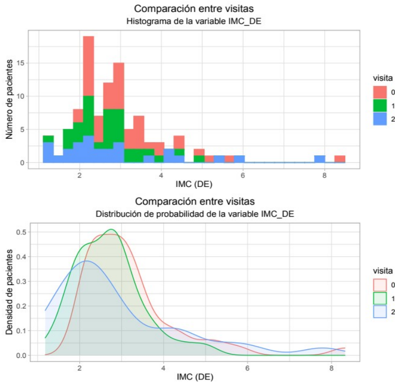
Figura 4.6: Histograma y densidad de la evolución del IMC en unidades DE
