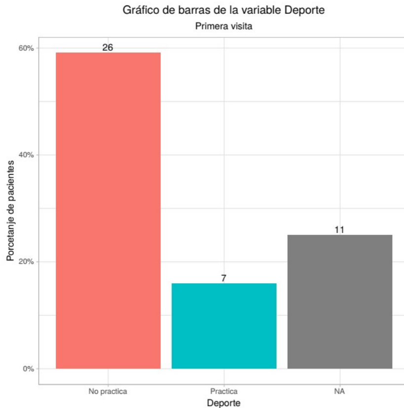
Figura 4.2: Gráfico de barras de la variable Deporte
