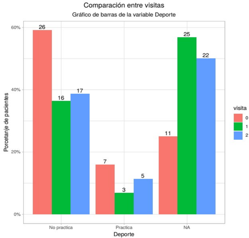
Figura 4.3: Evolución de la práctica de deporte entre visitas
