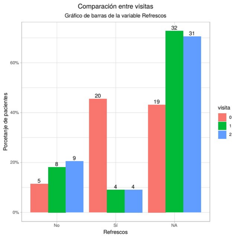
Figura 4.5: Evolución del consumo de refrescos entre visitas
