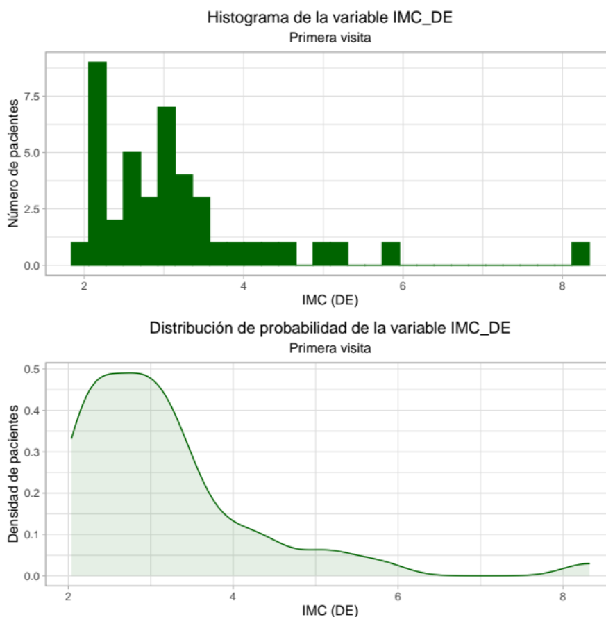
Figura 4.1: Histograma y distribución del IMC en unidades DE
