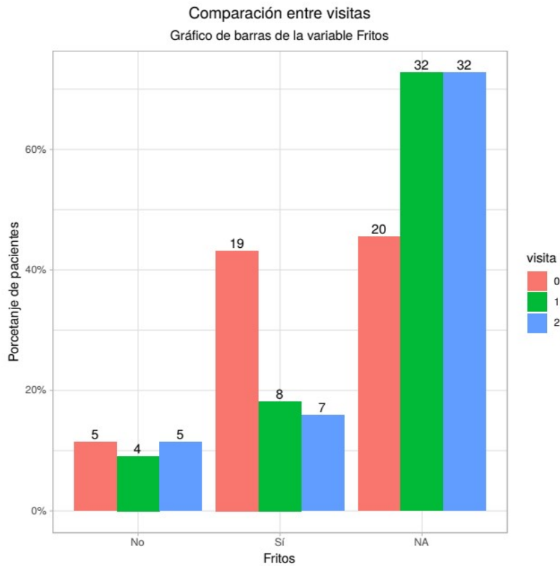
Figura 4.4: Evolución del consumo de fritos entre visitas
