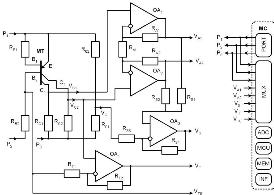
Рис. 10. Схема сигнального перетворювача мультифункціонального сенсора
