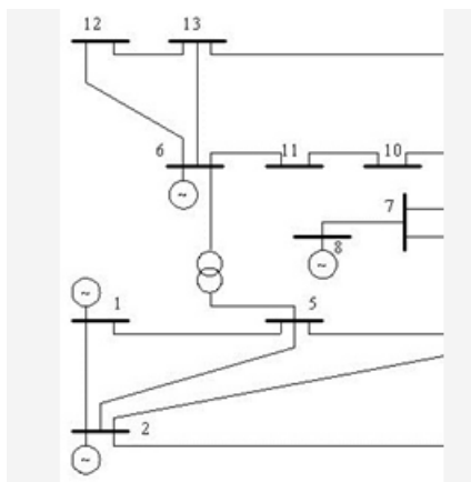
Рис.1. Тестова схема мережі на 14 вузлів - IEEE-14
