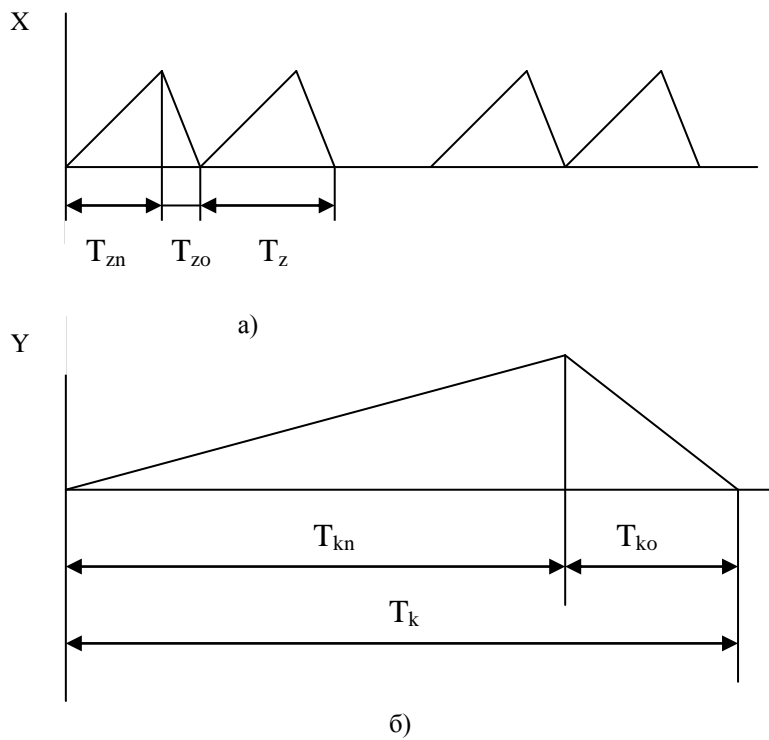
Рис. 5.2. Часові діаграми рядкової X та кадрової Y розгорток
