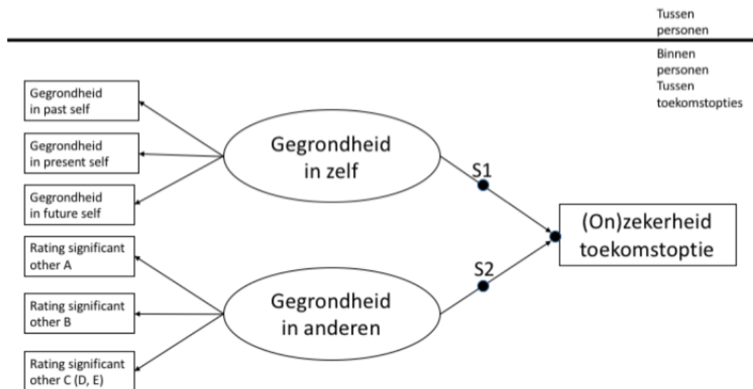
Figuur 1. Multilevel structural equation model (SEM) met een random intercept voor de (on)zekerheids-variabele, en random slopes (S1 en S2) voor de relaties tussen gegrontheid in zelfbeeld/anderen en (on)zekerheid op toekomstoptie-niveau (binnen personen).
