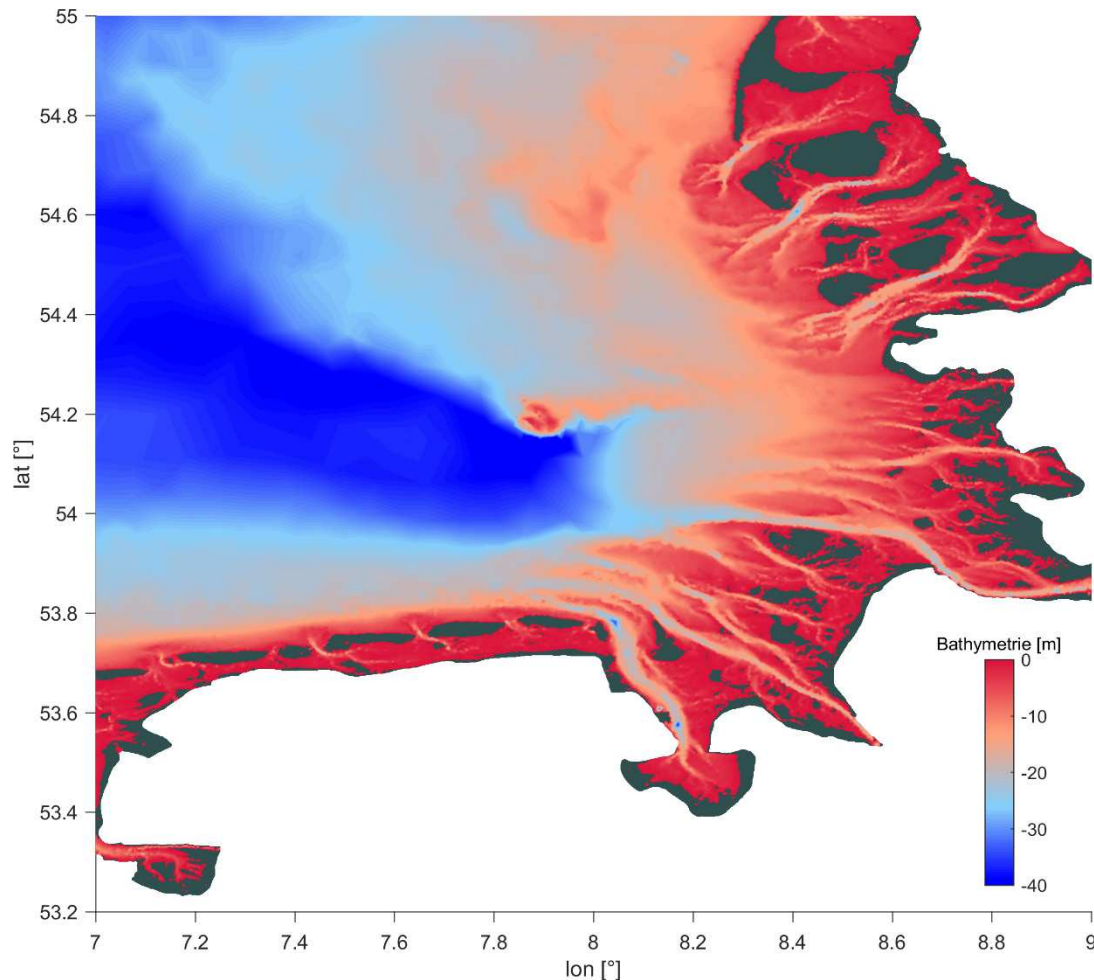
Abbildung 3: Zusammgeführte Höhenwerte der finalen Bathymetrie des HNMs als Konturplot (Ausschnitt). Zur besseren Differenzierung der Höhenwerte wurden alle Werte < -40 m in einer Farbe dargestellt und Werte > 0 m aus dem Datensatz eliminiert.
