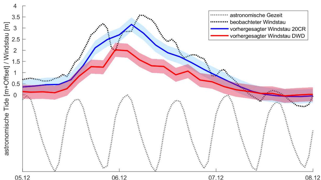
Abbildung 14: Vergleich der Rekonstruktion des Orkans „Xaver“ am Pegel Cuxhaven mit Reanalysedaten und DWD-Vorhersagen.
