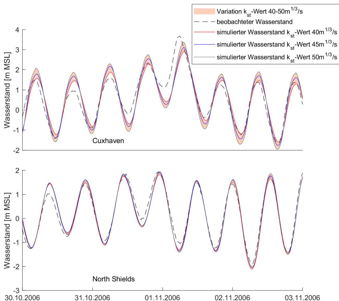
Abbildung 6: Einfluss der Rauheit auf die Wasserstände am Pegel Cuxhaven (oben) und North Shields (unten) zwischen dem 30.10.2006 und dem 03.11.2006 (Allerheiligenflut).
