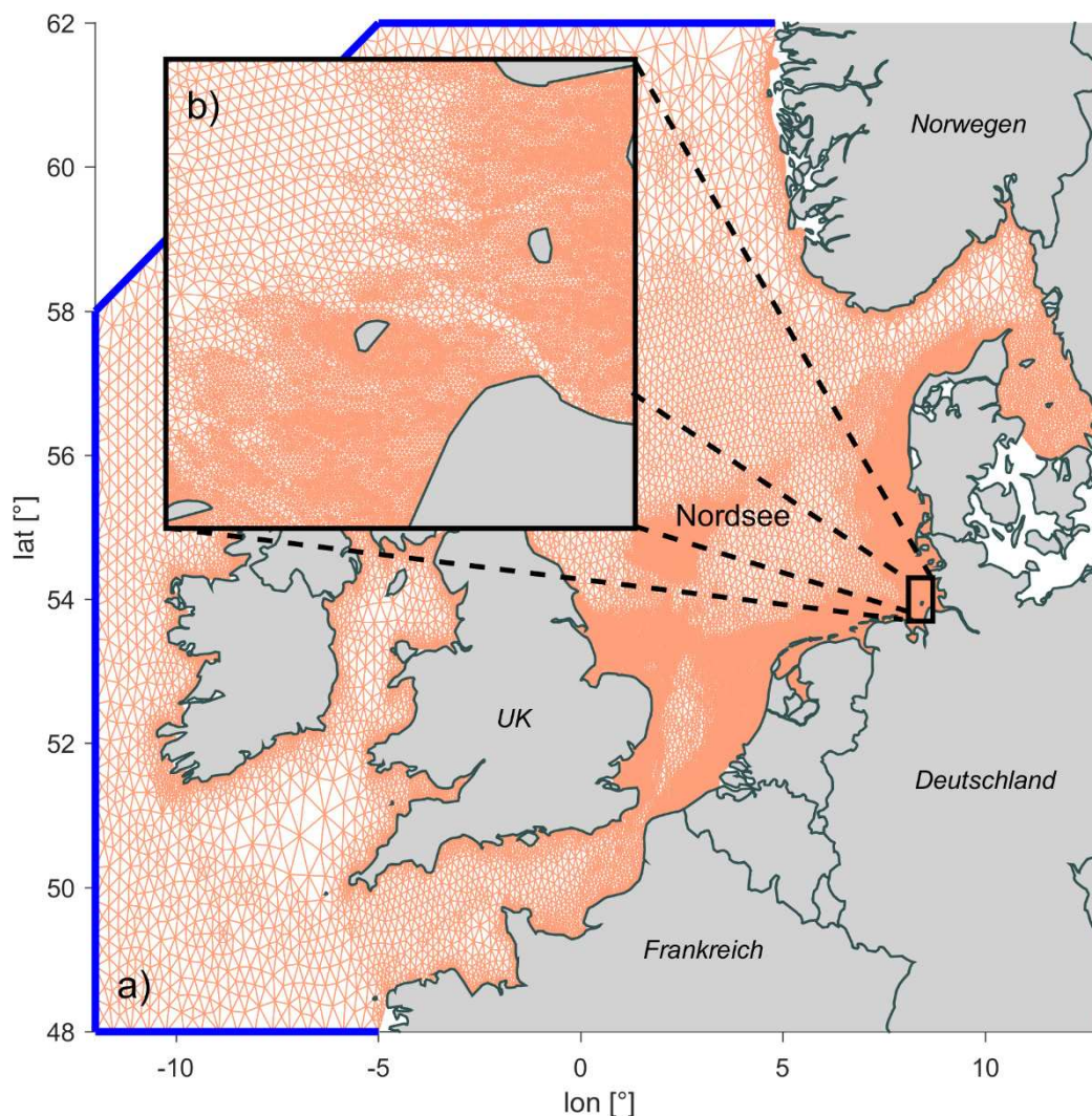
Abbildung 2: a) Modellgebiet und Rechengitter des HNMs. b) Detailausschnitt des Modellgebiets des Elbmündungsgebietes.
