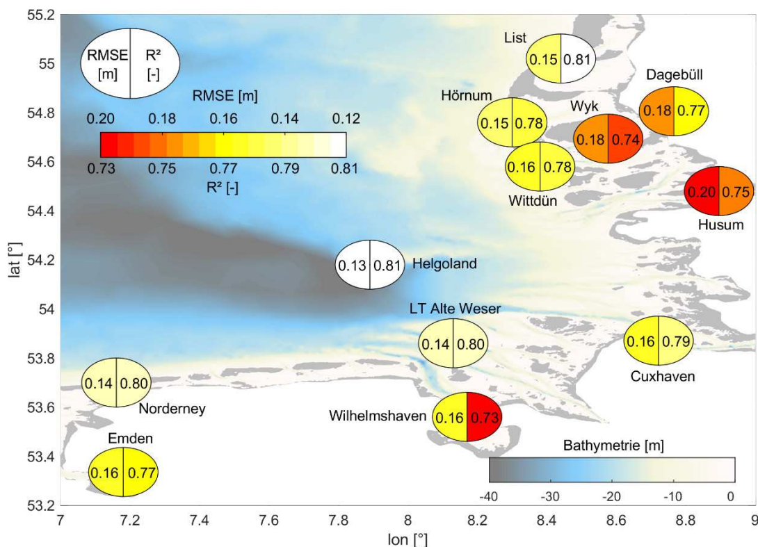
Abbildung 11: Effizienzkriterien der empirisch-statistischen Windstaumodelle (ohne Berücksichtigung der Interaktion zwischen Tide und Windstau) an den Pegelstandorten in der Deutschen Bucht.
