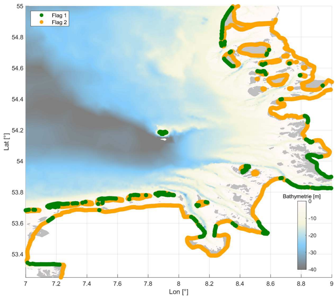
Abbildung 8: Exportierte Küstenlinie aus dem HNM (1.484 Punkte im Abstand von etwa 1 km) mit zugeordneten Flags.
