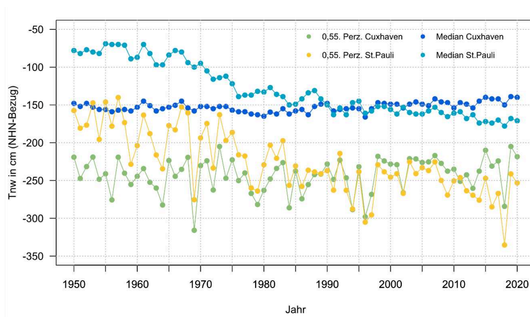
Abbildung 7-7 | Perzentile des Tnw der jeweiligen Jahre bei Cuxhaven und St. Pauli: 50. Perzentil: blau- St. Pauli , dunkelblau- Cuxhaven; 0,55. Perzentil (niedrigstes Tnw des jeweiligen Jahres): gelb - St. Pauli , grün: Cuxhaven.
