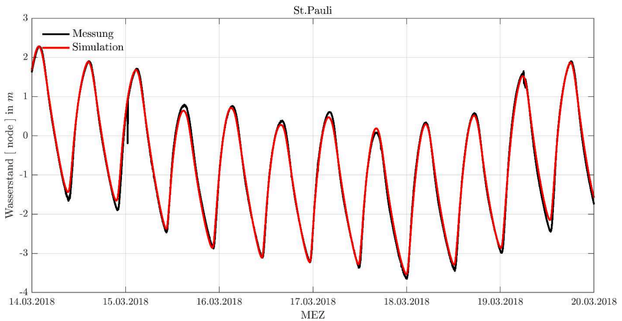
Abbildung 4-4 | Sturmebbe 2018, Wasserstandsentwicklung am Pegel St. Pauli, Messung (schwarz) und Simulationsergebnis (rot).
