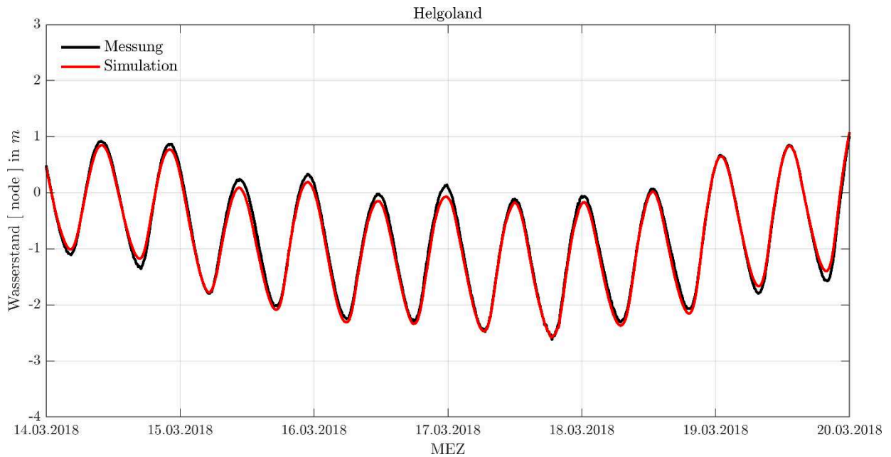
Abbildung 14-1 | Sturmebbe 2018, Wasserstandsentwicklung am Pegel Helgoland, Messung (schwarz) und Simulationsergebnis (rot).
