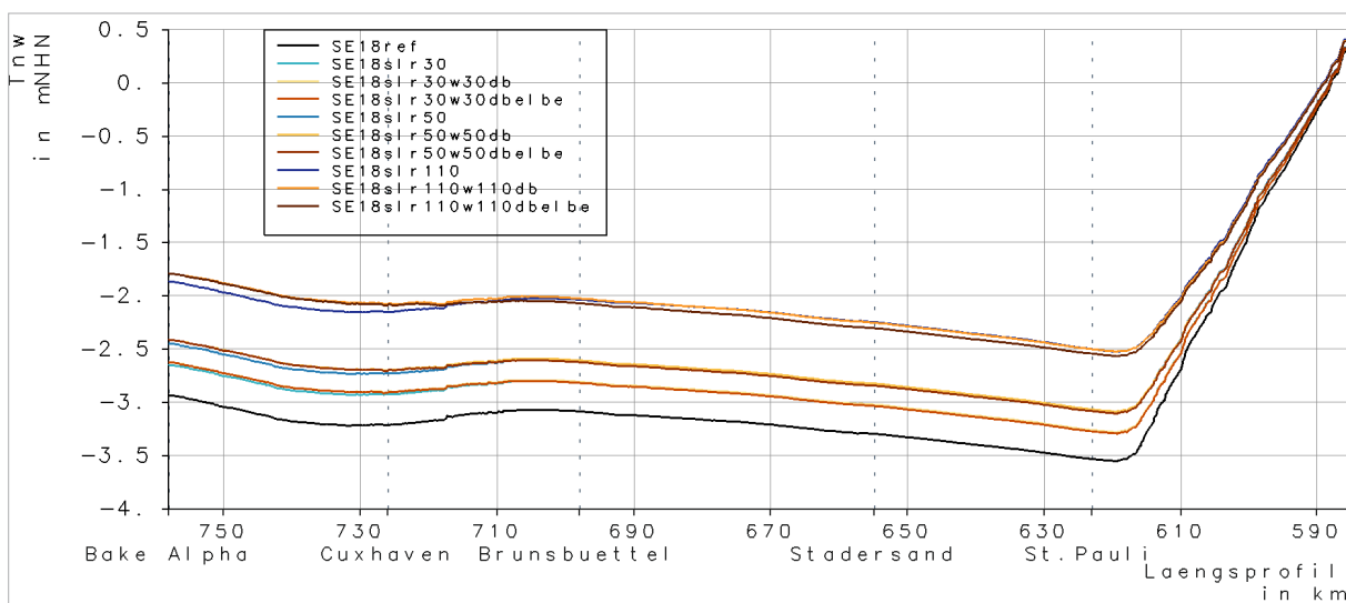
Abbildung 9-11 | Sturmflut 2018: NTnw entlang der Tideelbe ohne SLR (schwarz), und bei verschiedenen SLR- und Wattwachstumsszenarien.
