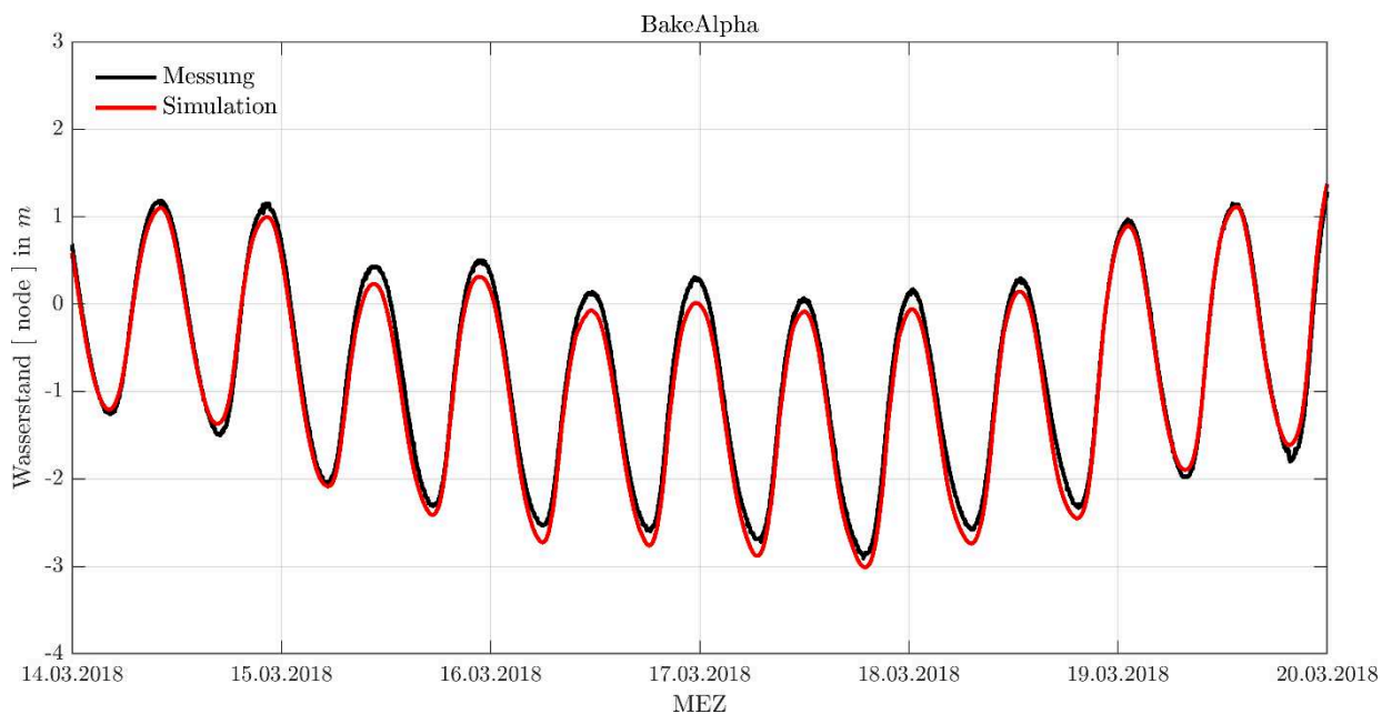
Abbildung 14-2 | Sturmebbe 2018, Wasserstandsentwicklung am Pegel Bake Alpha, Messung (schwarz) und Simulationsergebnis (rot).
