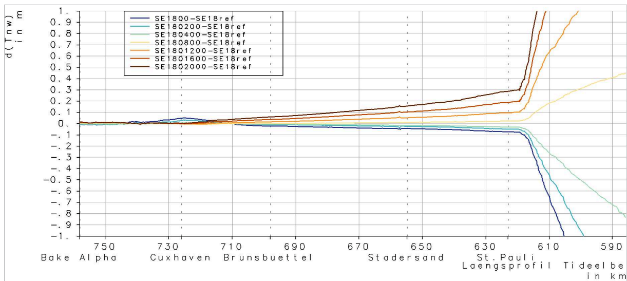
Abbildung 9-2 | Sturmebbe 2018: Änderung des NTnw entlang der Tideelbe relativ zum Referenzabfluss (600-700 m 3 /s) bei variiertem Abfluss.
