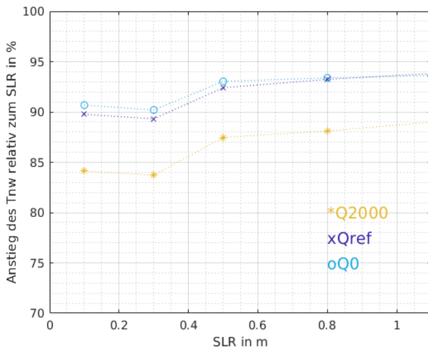
Abbildung 9-9 | Sturmebbe 2018: Änderung des NTnw am Pegel St. Pauli bei verschiedenen Meeresspiegelanstiegsszenarien bei Referenzabfluss (lila) sowie bei einem Abfluss von 0 (blau) und 2000 m 3 /s (gelb).
