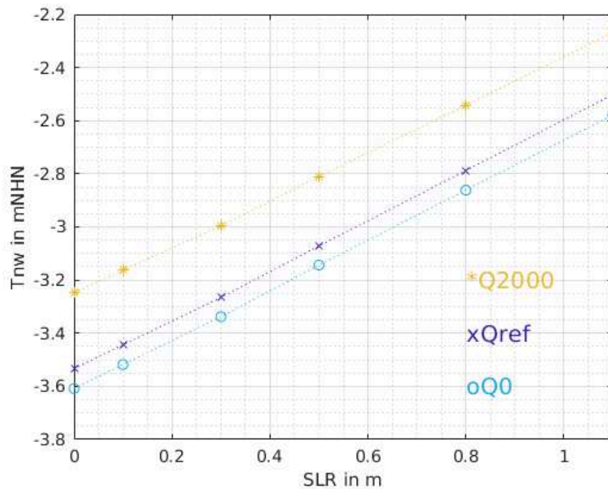
Abbildung 9-8 | Sturmebbe 2018: NTnw am Pegel St. Pauli bei verschiedenen Meeresspiegelanstiegsszenarien bei Referenzabfluss (lila) sowie bei einem Abfluss von 0 (blau) und 2000 m 3 /s (gelb).
