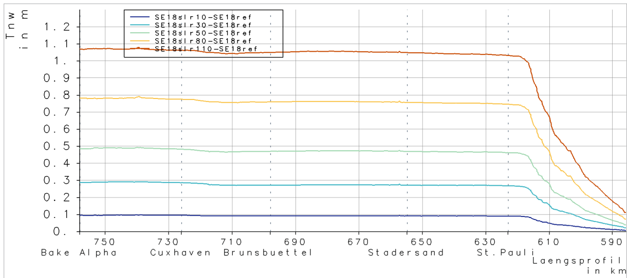
Abbildung 9-7 | Sturmeebe 2018: Änderung des niedrigstes NTnw entlang der Tideelbe zum Referenzzustand ohne SLR bei verschiedenen SLR-Szenarien mit Referenzabfluss.
