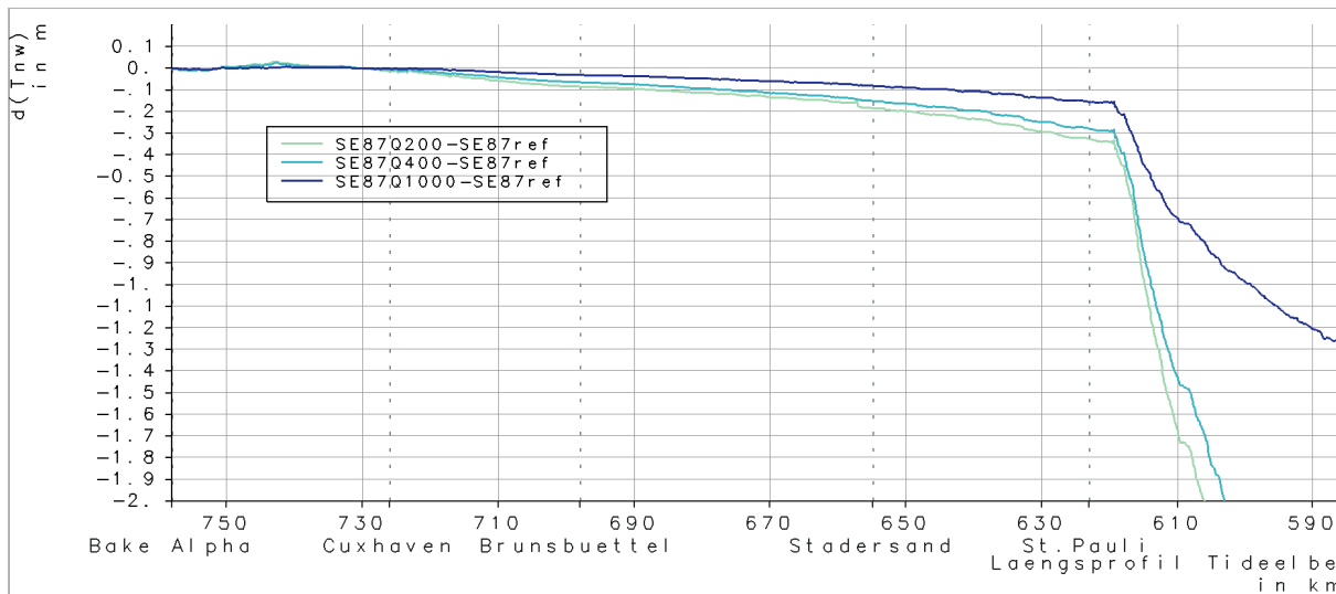
Abbildung 9-17 | Sturmflut 1987: Differenz des NTnw der Sturmflut 1987 entlang der Tideelbe zum Szenario mit gemessenem Abfluss ( 1600\text{m}^3/\text{s} ): blau: Simulationsergebnis bei einem Abfluss von 400\text{m}^3/\text{s} , grau: Simulationsergebnis bei einem Abfluss von 200\text{m}^3/\text{s} .
