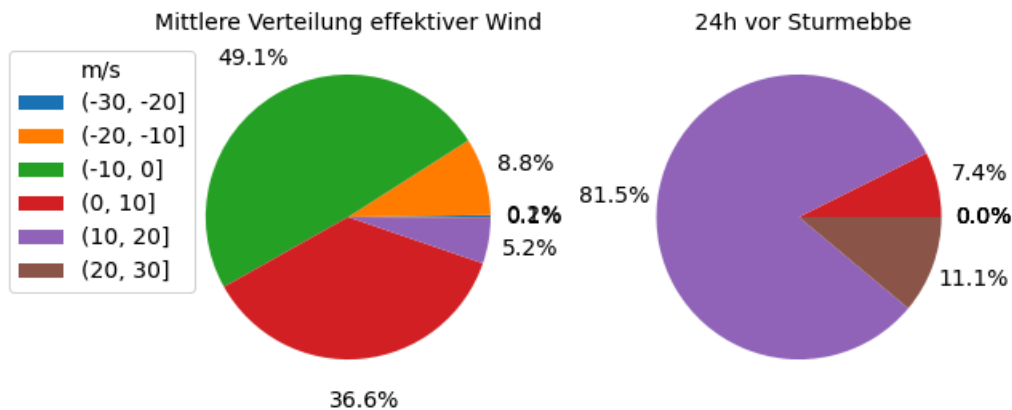
Abbildung 6-5 | Links: Mittlere Verteilung des effektiven Windes aus der LAMB-Wetterlagenklassifikation projiziert auf 142° eingeteilt in 10 m/s Klassen, ermittelt aus Tagesmitteln des ERA5 Luftdrucks auf Meeresniveau für den gesamten untersuchten Zeitraum von 1950 bis 2019. Rechts: Mittlere Verteilung des effektiven Windes aus der LAMB-Wetterlagenklassifikation projiziert auf 142° eingeteilt in 10 m/s Klassen 24 Stunden vor den Sturmeebben am Pegel Cuxhaven (Tnw unter 0,55. Perzentil aller Tnw) zwischen 1950 und 2019.
