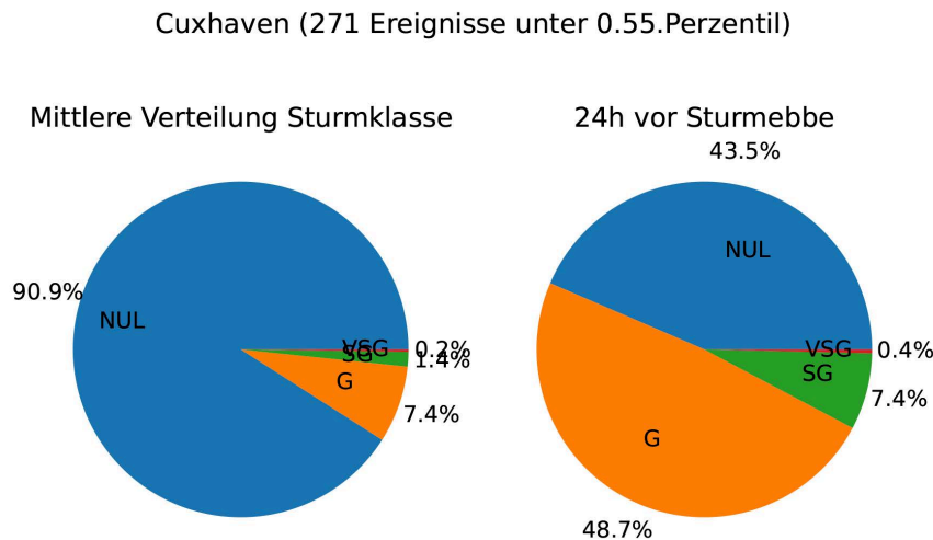
Abbildung 6-2 | Links: Mittlere Verteilung der LAMB Sturmklassen, ermittelt aus Tagesmitteln des ERA5 Luftdrucks auf Meeresebene für den gesamten untersuchten Zeitraum von 1950 bis 2019. Rechts: Mittlere Verteilung der LAMB Sturmklassen 24 Stunden vor den Sturmebben am Pegel Cuxhaven (Tnw unter 0,55. Perzentil aller Tnw) zwischen 1950 und 2019.
