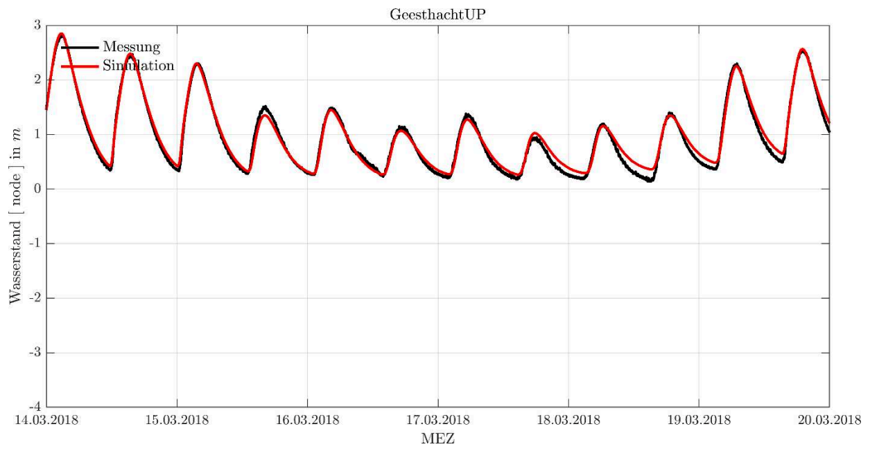
Abbildung 14-7 | Sturmeebe 2018, Wasserstandsentwicklung am Pegel Geesthacht UP, Messung (schwarz) und Simulationsergebnis (rot)
