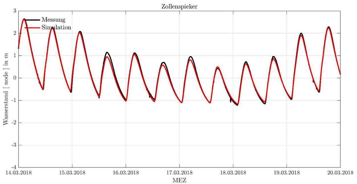
Abbildung 14-6 | Sturmeebe 2018, Wasserstandsentwicklung am Pegel Zollenspieker, Messung (schwarz) und Simulationsergebnis (rot).
