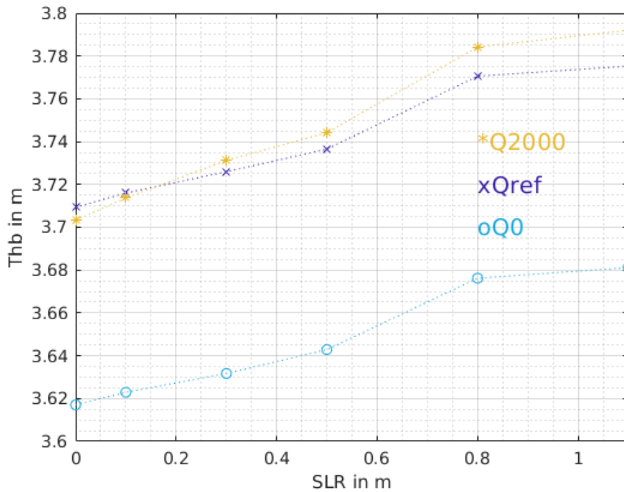
Abbildung 9-10 | Sturmflut 2018: Thb der niedrigsten Tide am Pegel St. Pauli bei verschiedenen Meeresspiegelanstiegsszenarien bei Referenzabfluss (lila) sowie bei einem Abfluss von 0 (blau) und 2000 m³/s (gelb).
