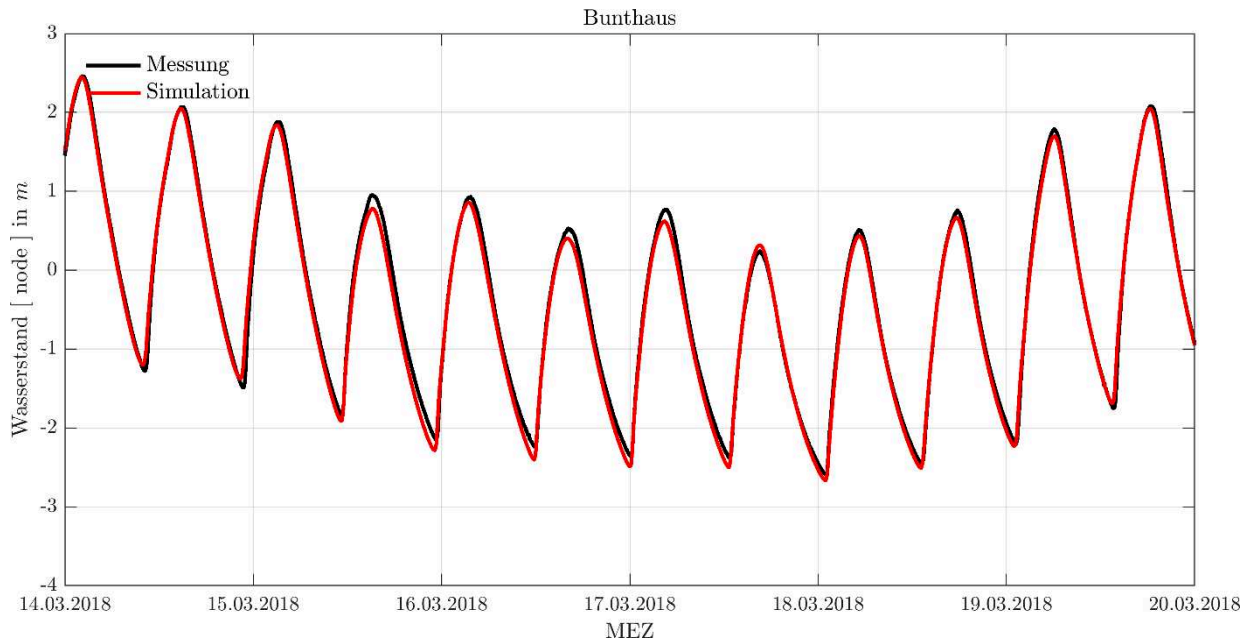
Abbildung 14-5 | Sturmeebe 2018, Wasserstandsentwicklung am Pegel Bunthaus, Messung (schwarz) und Simulationsergebnis (rot).
