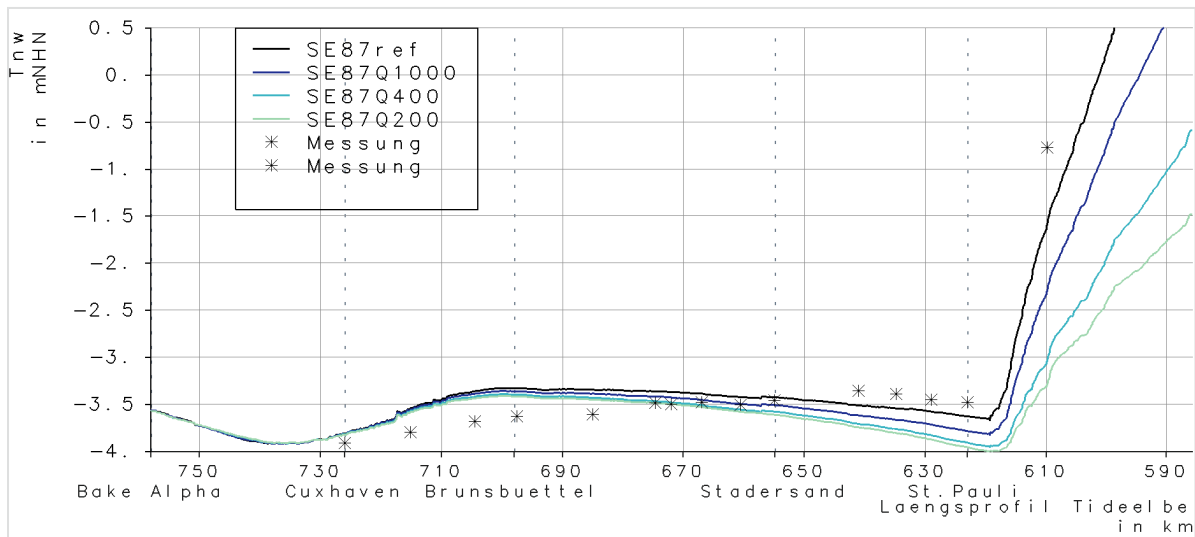
Abbildung 9-16 | Sturmebbe 1987: NTnw der Sturmebbe 1987 entlang der Tideelbe: grün: Simulationsergebnis bei gemessenem Abfluss (ca. 1600 \text{ m}^3/\text{s} ), blau: Simulationsergebnis bei einem Abfluss von 400 \text{ m}^3/\text{s} , grau: Simulationsergebnis bei einem Abfluss von 200 \text{ m}^3/\text{s} , schwarze Marker: Messung.
