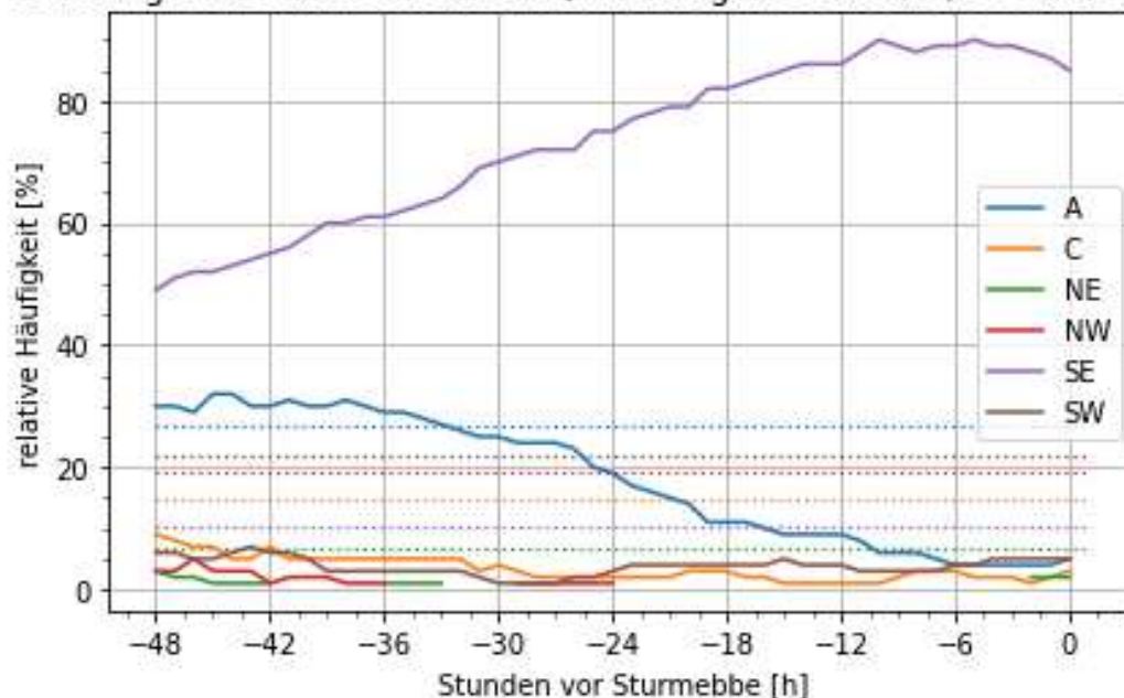
Abbildung 6-6 | Verteilung der LAMB Wetterlagen aus ERA5 in den 48 Stunden vor dem Tnw. Die gepunktete Linie kennzeichnet die mittlere Häufigkeit der jeweiligen Wetterlage im Zeitraum 1950–2019.
