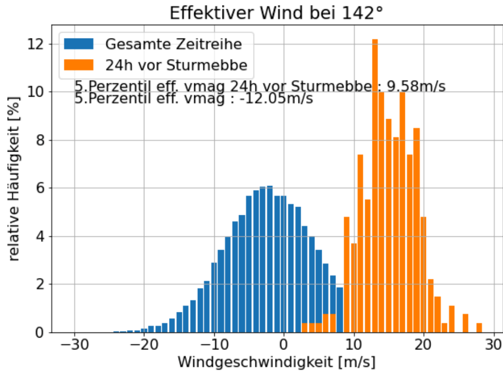
Abbildung 6-4 | Verteilung des effektiven Windes projiziert auf 142° über die Tagesmittel des gesamten Zeitraumes 1950–2019 (blau) und im 24-Stunden-Mittel vor den 271 Sturmeebben(orange). Außerdem dargestellt ist das 5. Perzentil des effektiven Windes der beiden Datensätze.
