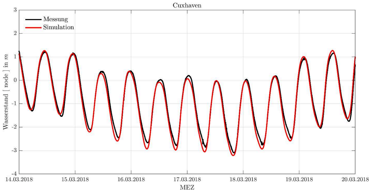
Abbildung 4-3 | Sturmebbe 2018, Wasserstandsentwicklung am Pegel Cuxhaven, Messung (schwarz) und Simulationsergebnis (rot).
