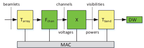
Fig. 28. Apertif correlator subsystem.
