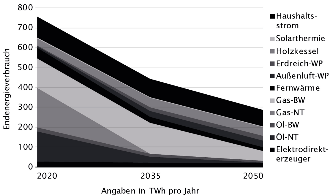
Abb. 5.18 Mögliche zukünftige Anteile der Wärmeerzeuger und des Haushaltsstroms am Endenergieverbrauch des Wohngebäudesektors (ohne Neubau) in Deutschland (moderater Elektropfad)
