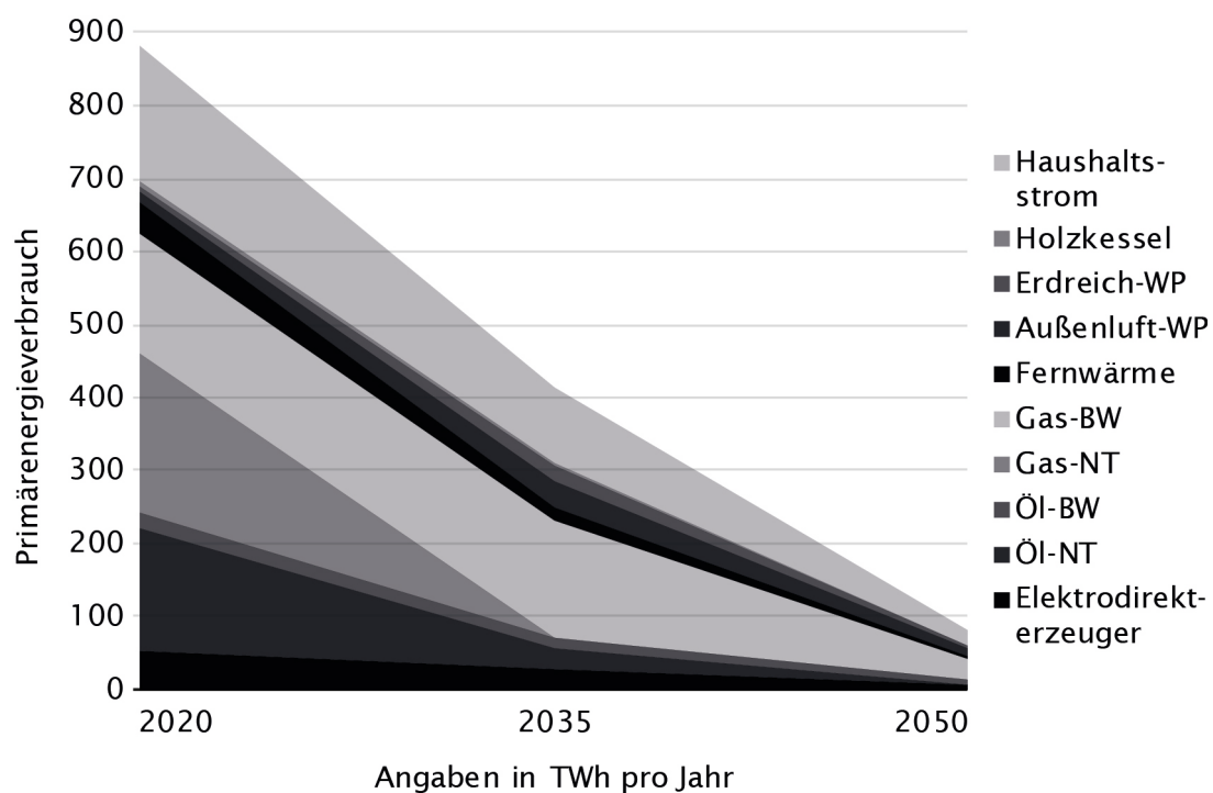
Abb. 5.20 Mögliche zukünftige Anteile der Wärmeerzeuger und des Haushaltsstroms am Primärenergieverbrauch des Wohngebäudesektors (inklusive Neubau) in Deutschland (moderater Elektropfad)
