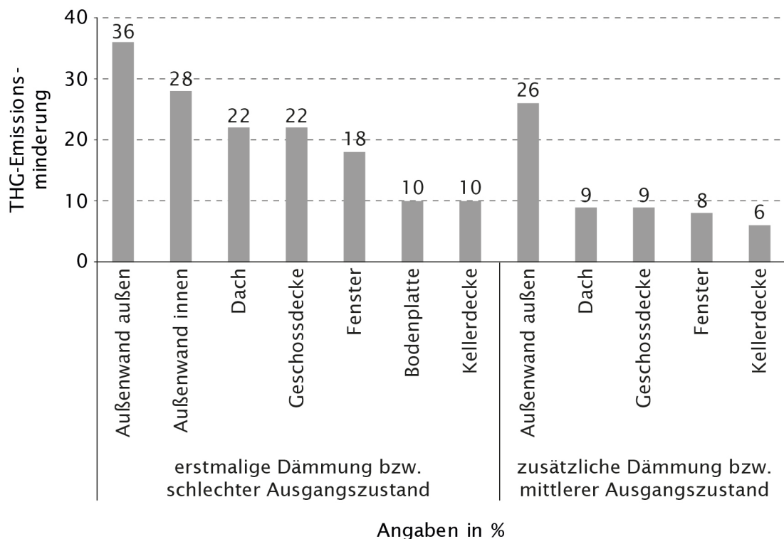
Abb. 4.10 THG-Emissionsminderungen von Sanierungsmaßnahmen an der Gebäudehülle bei einem durchschnittlichen Mehrfamilienhaus
