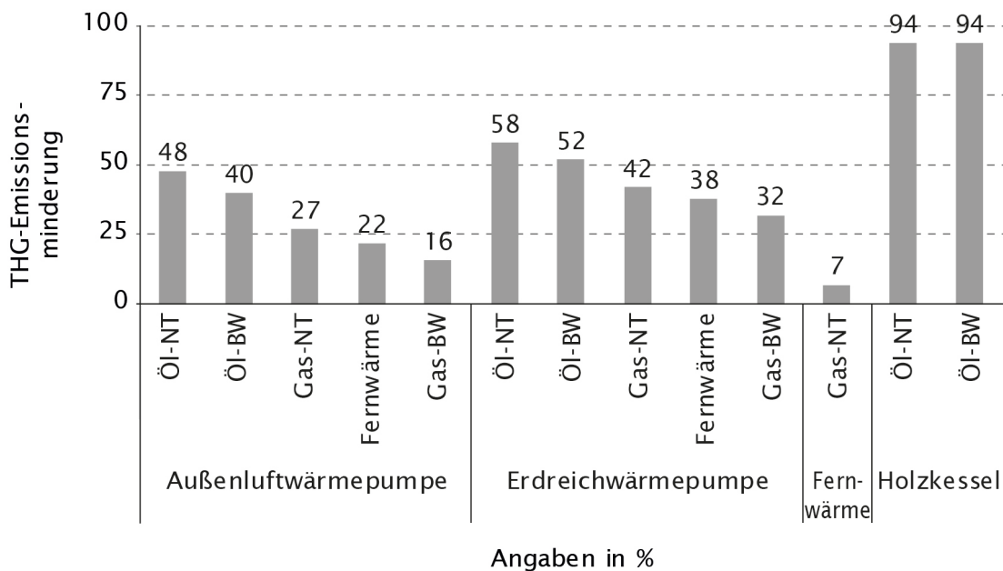
Abb. 4.2 THG-Emissionsminderung durch Austausch eines Heizkessels mit fossilen Brennstoffen durch eine Wärmepumpe, Fernwärme oder einen Holzkessel bei einem durchschnittlichen Mehrfamilienhaus
