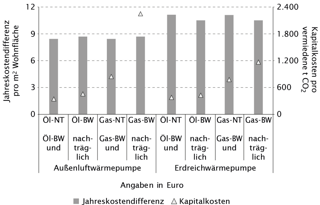
Abb. 4.13 Jahreskostendifferenz und Kapitalkosten pro vermiedener t CO 2 für Heizungshybridssysteme bei einem durchschnittlichen Ein- bzw. Zweifamilienhaus
