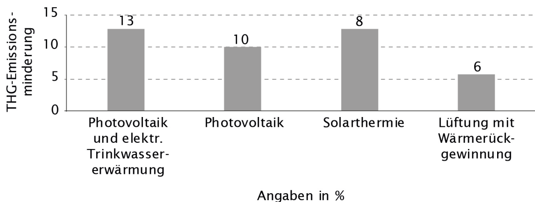
Abb. 4.4 THG-Emissionsminderung durch zusätzliche Erzeuger bei einem durchschnittlichen Mehrfamilienhaus
