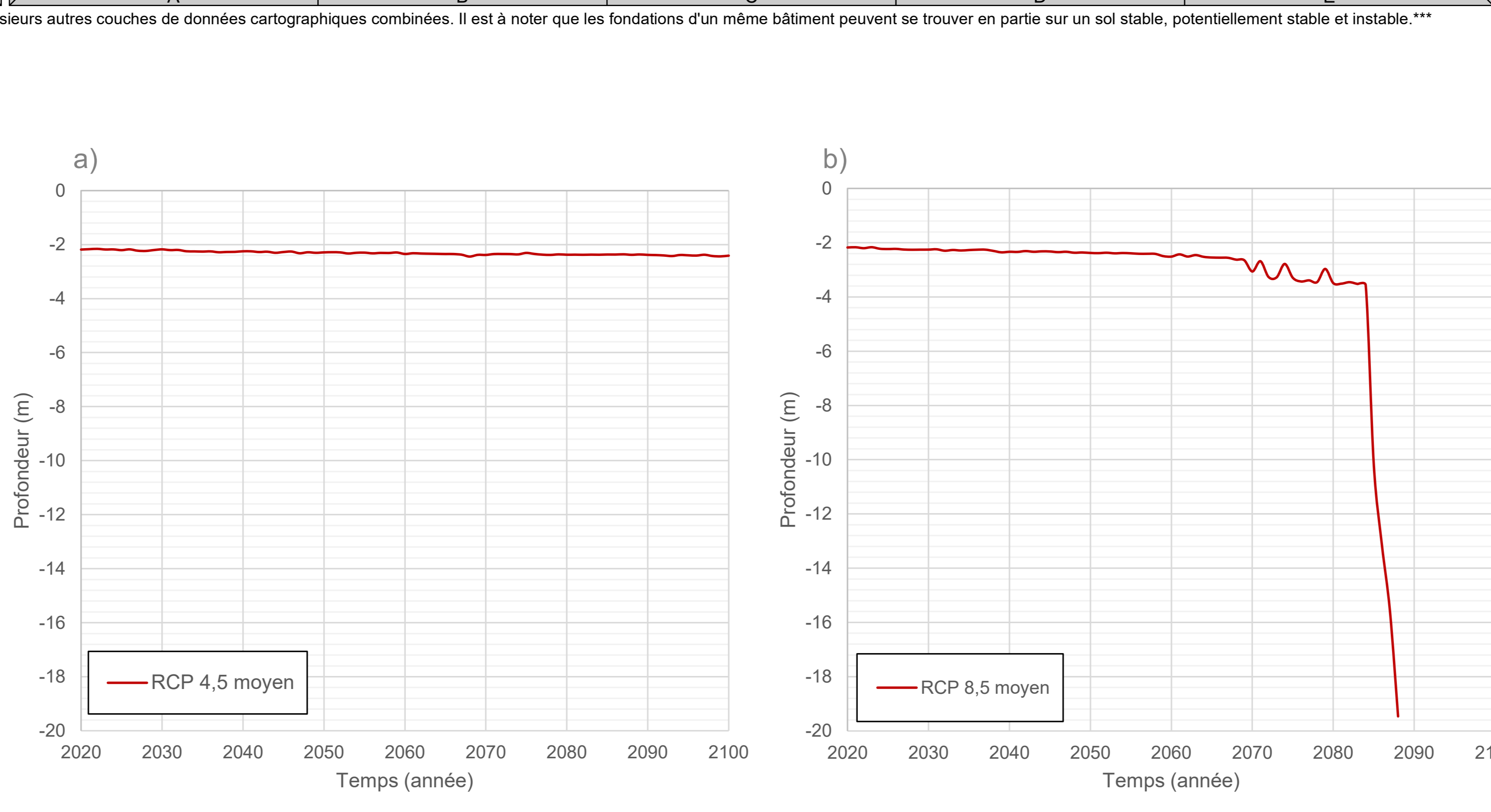
Figure 2 : Évolution de l'épaisseur de la couche active à partir du modèle MRCC5 selon les scénarios a) RCP 4,5 moyen d'augmentation de gaz à effet de serre, b) RCP 8,5 moyen d'augmentation de gaz à effet de serre pour le modèle HT-156 de 2020 à 2100.
