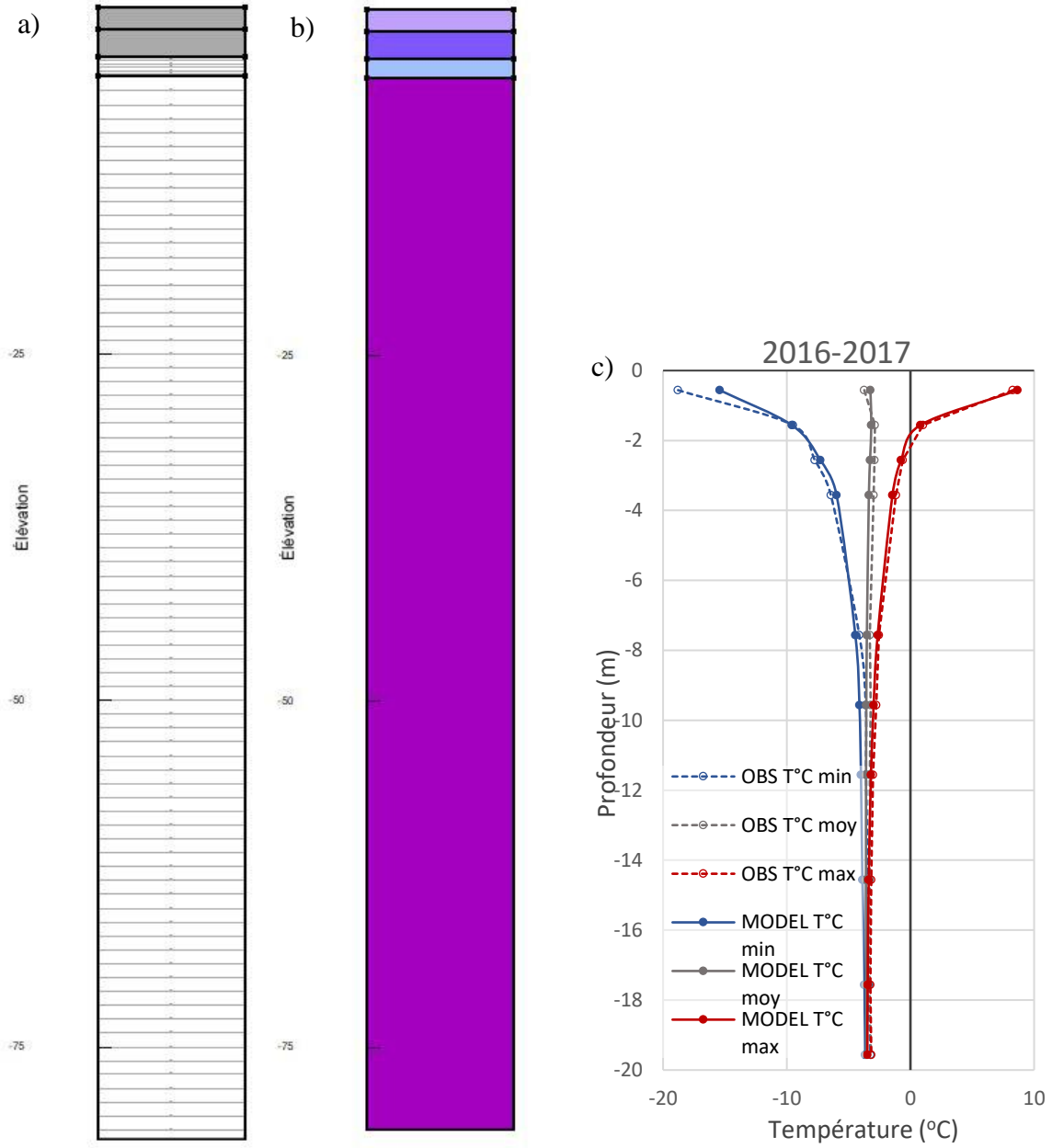
Figure 21 : a) Maillage, b) géométrie et conditions limites, ainsi que c) propriétés géothermiques du modèle théorique, localisé dans des sables et graviers, à l'aéroport de Quaqtaq.
