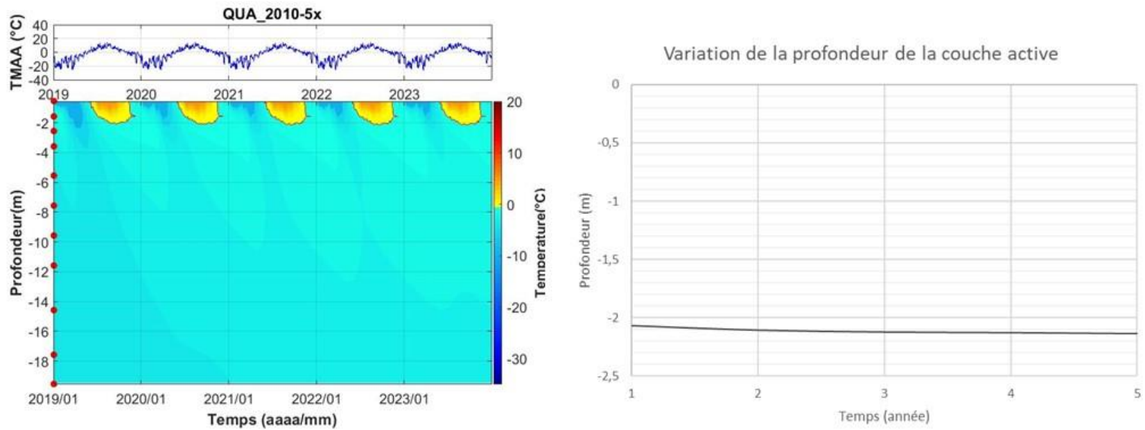
Figure 24 : Variation de la température du pergélisol et de la profondeur de la couche active, soumise à une série de 5x les températures observées durant l'année 2009-2010, pour le modèle HT-156
