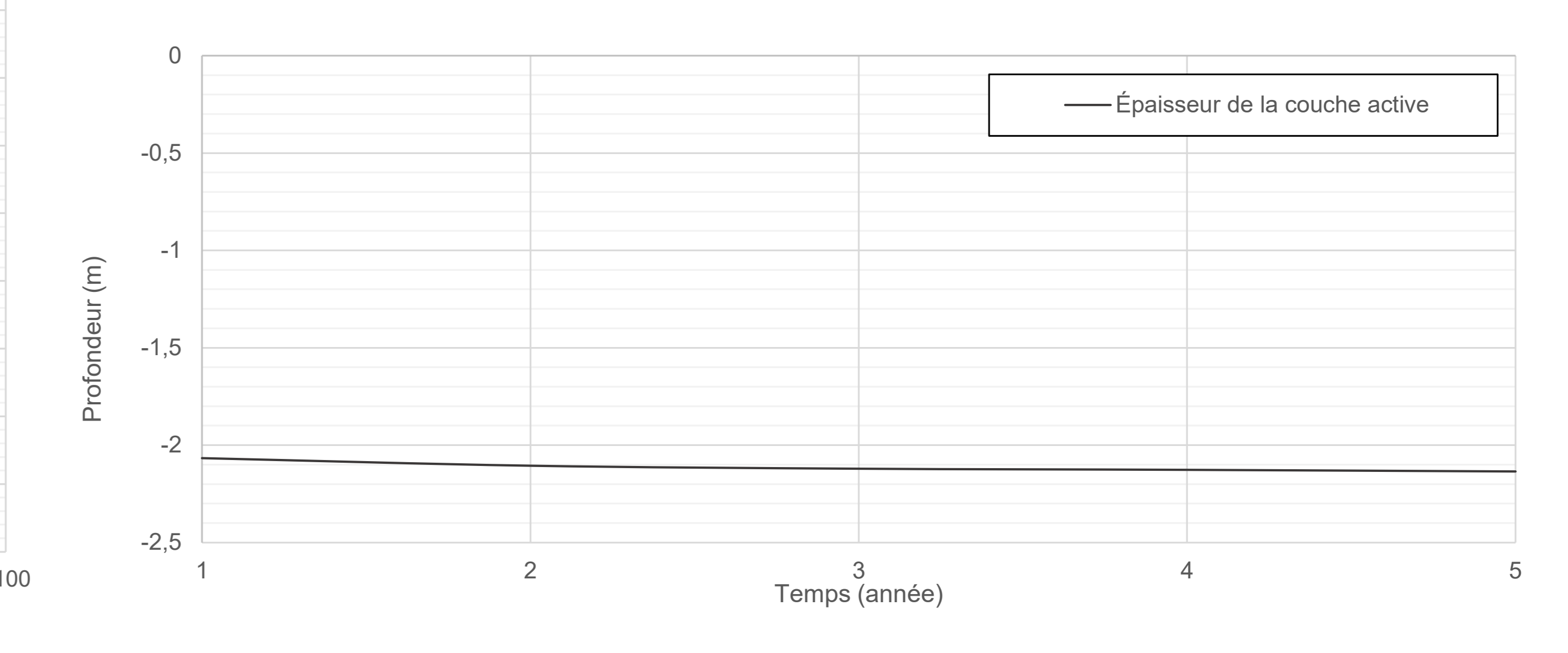
Figure 3 : Variation de la température du pergélisol et de l'épaisseur de la couche active, soumise à une série de 5x les températures observées durant l'année climatique de 2009-2010 pour le modèle HT-156, situé en terrain naturel à proximité de l'aéroport. À l'endroit de la station, cinq années chaudes consécutives auraient un impact limité sur l'approfondissement de la couche active.
