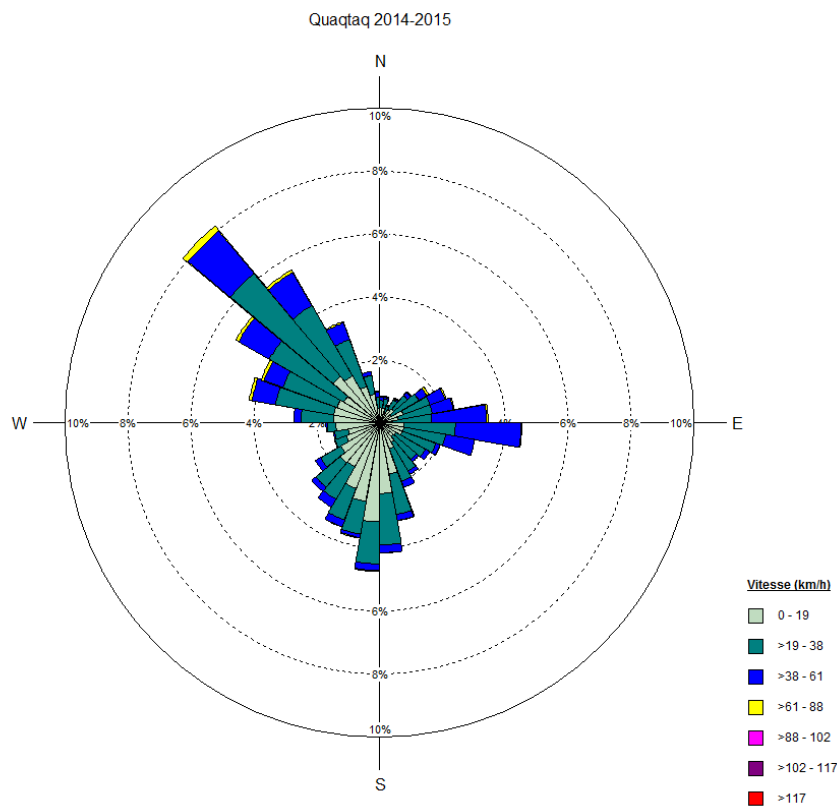
Figure 18 : Moyenne horaire de la direction et de la vitesse des vents selon l'échelle de Beaufort pour la période de 2014 à 2015 à la station d'Environnement Canada à Quaqtaq
