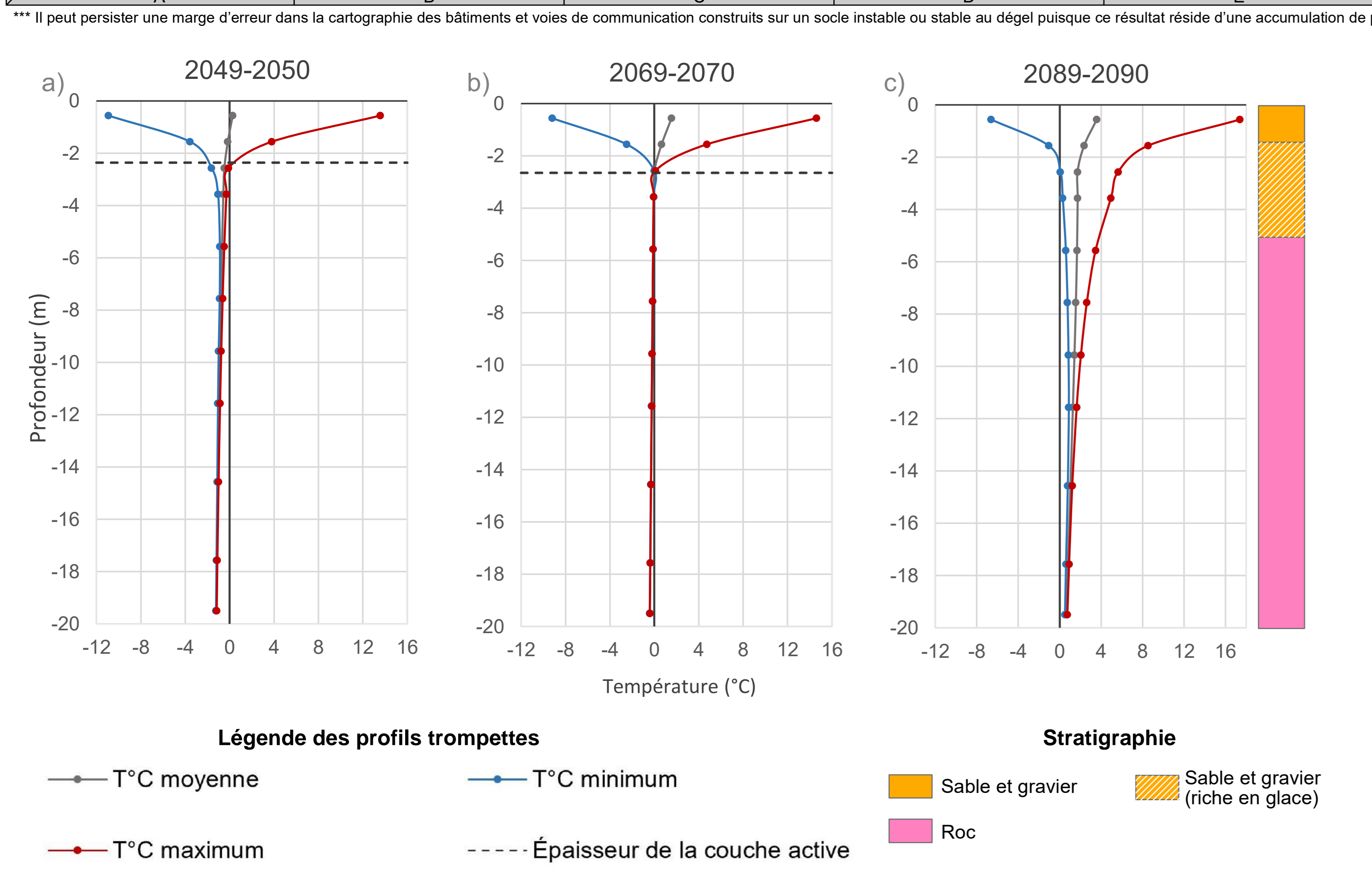
Figure 1 : Profils de la température projetée moyenne, minimum et maximum du sol pour la station HT-156 selon le scénario RCP 8.5. a) L'épaisseur maximale atteinte par la couche active pour l'année climatique 2049-50, b) pour l'année climatique 2069-70 et c) celle de 2089-90. Entre les années 2070 et 2089, le dégel du sol dépasse les 20 mètres de profondeur.
