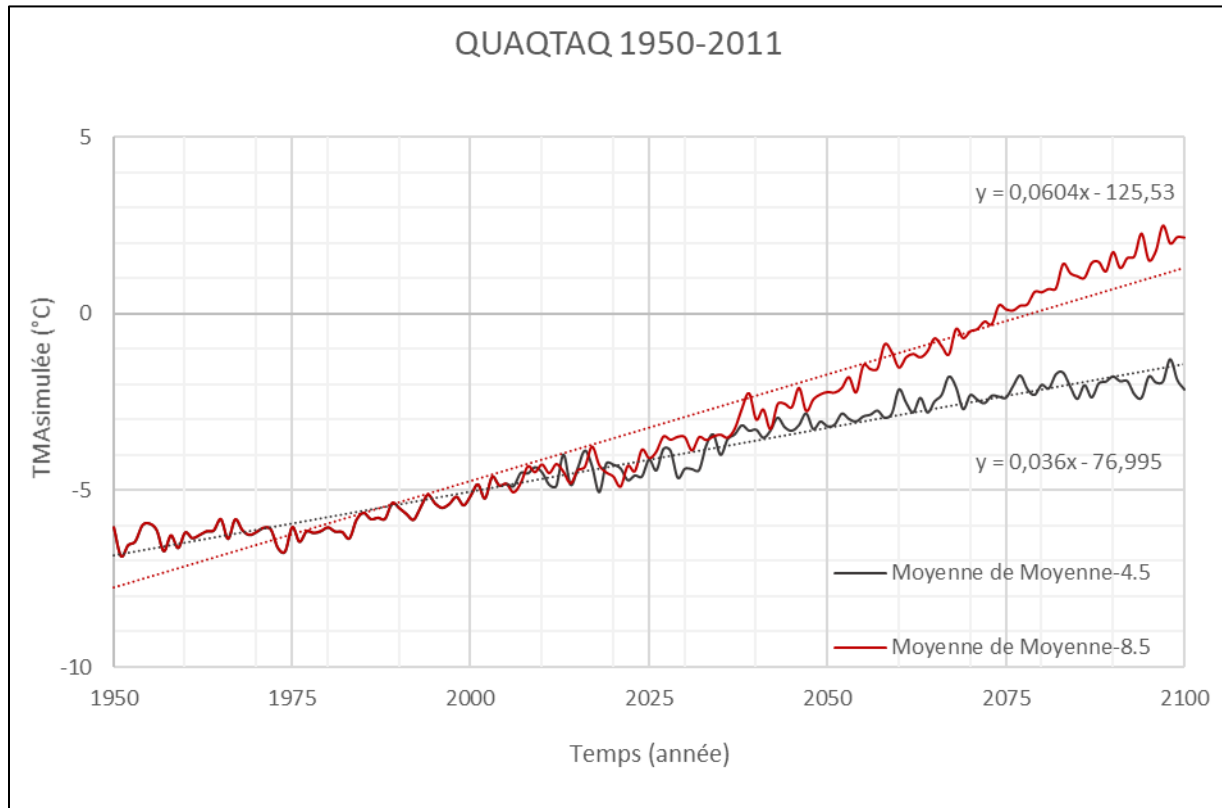
Figure 20 : Température moyenne annuelle de l'air (TMAA) simulée à partir de 10 sorties du modèle MRCC5 selon les scénarios 4.5 et 8.5 d'augmentation de gaz à effet de serre pour Quaqtac de 1950 à 2100.
