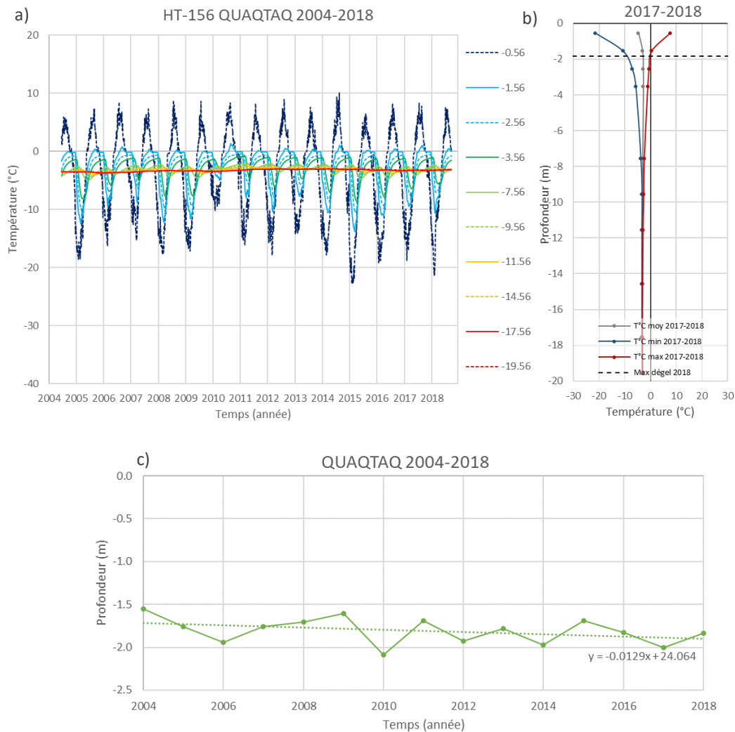
Figure 19 : a) Température du sol en fonction de la profondeur et du temps pour la période de 2004 à 2018, b) enveloppe de la température minimale, maximale et la moyenne annuelle 2017-2018 et c) profondeur maximale atteinte par le front de dégel pour la période de 2004 à 2018, enregistré au câble HT-156, dans le sable et gravier littoraux sur roc de l'aéroport de Quaqtaq.
