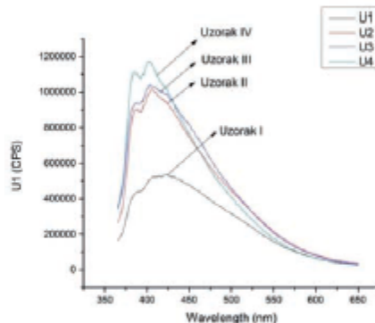
Slika 1. Fluorescentni spektri uzorka humniskih kiselina iz halde II
