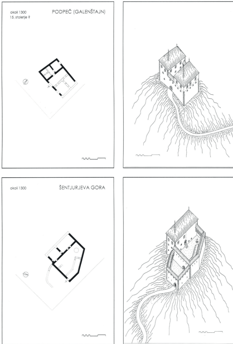
Slika 39. Gallenstein in Šentjurjeva gora, tloris in aksonometrična študija (avtor Igor Sapač).
