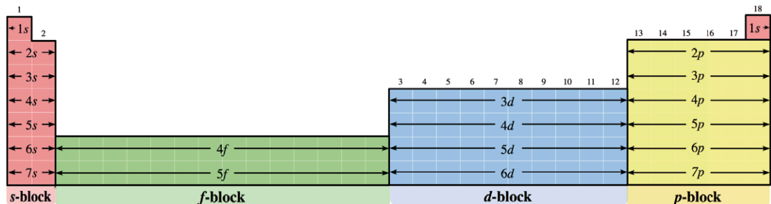
Fig. 3.5 – Tavola periodica degli elementi estesa, con indicazione dei blocchi relativi al riempimento degli orbitali atomici. [CC BY-SA 3.0]
