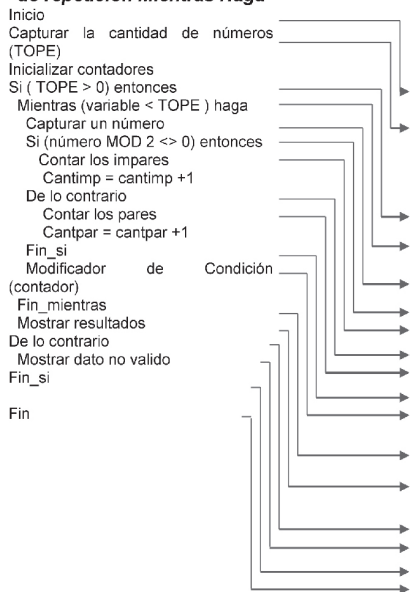
Figura 4.31 Relación entre el algoritmo y el pseudocódigo del ejemplo.
