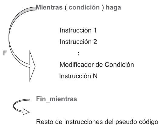
Figura 4.3 Funcionamiento de la estructura de repetición Mientras Haga cuando la condición da falso.
