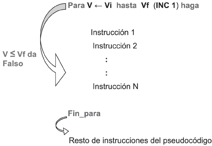
Figura 4.15 Funcionamiento de la estructura de repetición Para usando INC cuando V \leq V_f da falso.
