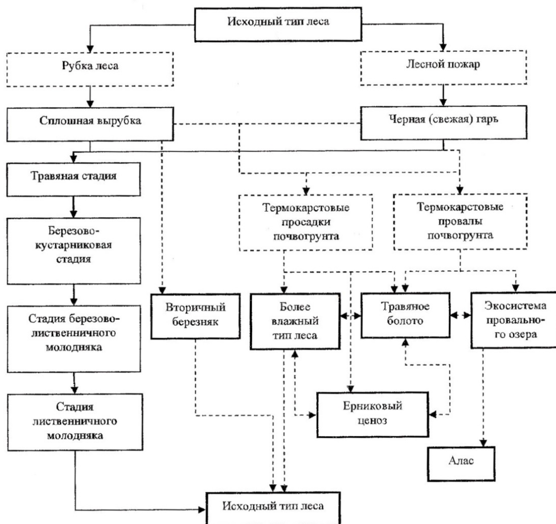
Рис. 1. Схема лесовозобновительной сукцессии в современных лиственничных лесах Якутии [3] Fig. 1. Scheme of reforestation succession in modern larch forests of Yakutia [3]
