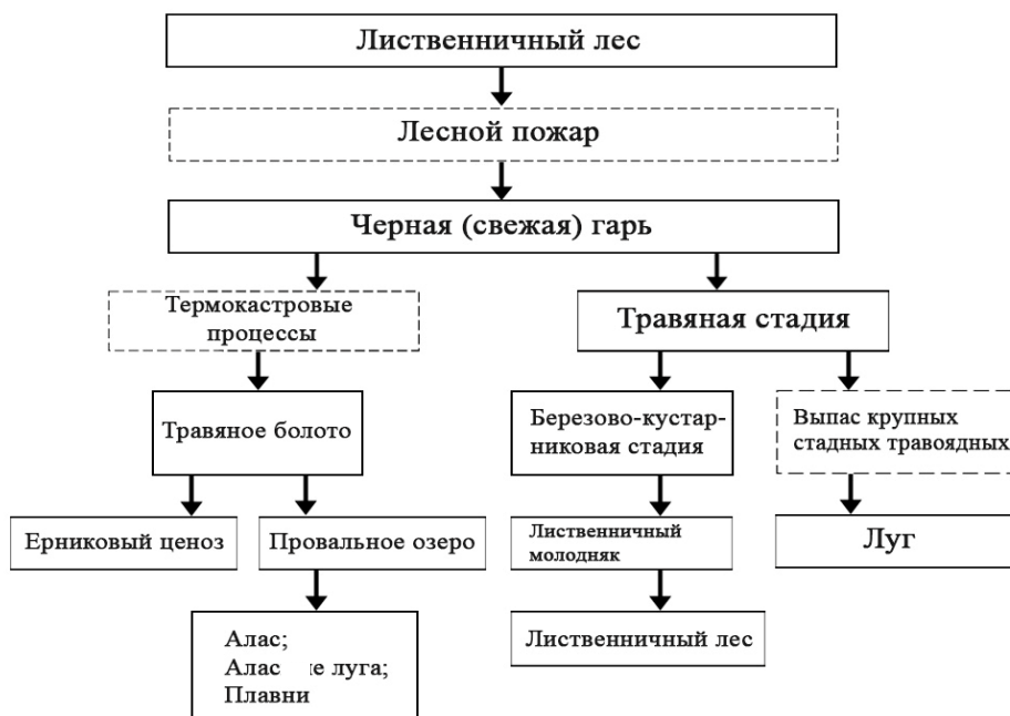
Рис. 2. Постпирогенный сукцессионный процесс позднего плейстоцена Fig. 2. Post-pyrogenic Late Pleistocene Succession Process
