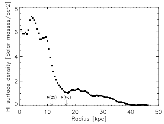
Fig. 13. Radial HI profile for NGC 5055. The arrows show the De Vaucouleurs ( R_{25} ) and Holmberg radii ( R_{Ho} ).
