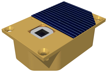
Fig. 2 Autonomous Sun Sensor (© TNO).
