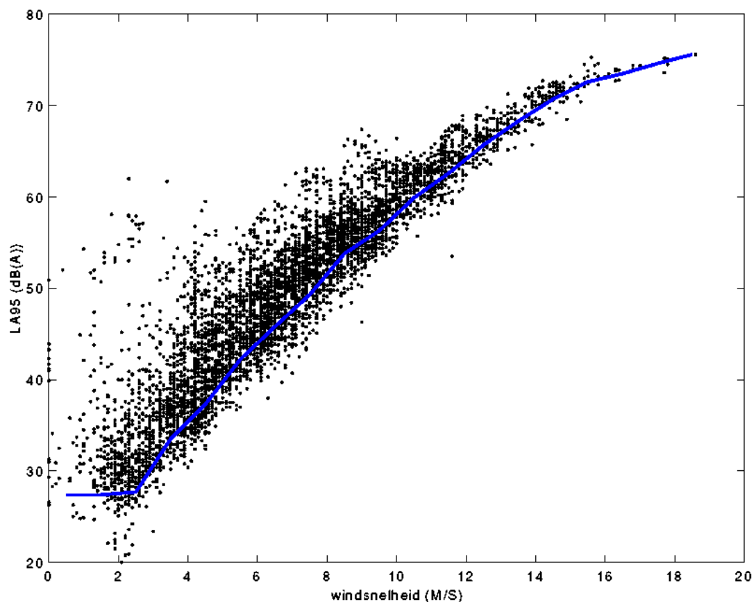
Figure 3.2: het achtergrondgeluidsniveau ( L_{A95} ) uitgezet tegen de windsnelheid. op 10 meter hoogte en over de gehele meetperiode. Elk punt in de wolk (totaal: ruim 5300 punten) representeert een meetblok van 10 minuten. De lijn verbindt punten waarbij alle meetblokken in klassen van 1 m/s zijn verdeeld.
